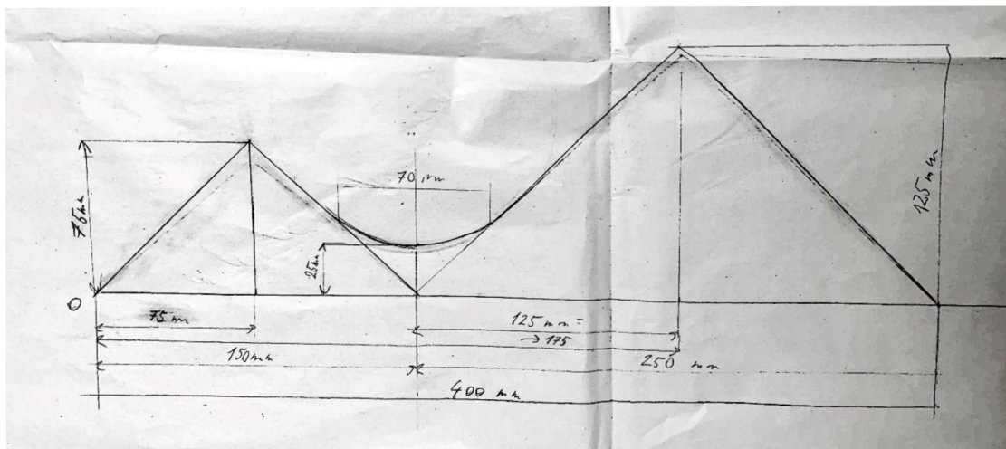
Obr. 22 Technický náčrtek řezu vertikální polovinou modelu, okótovaný [35]
