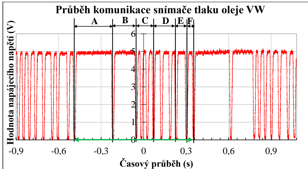
Obrázek 32: Průběh signálu SENT komunikace snímače tlaku oleje a jeho popis
