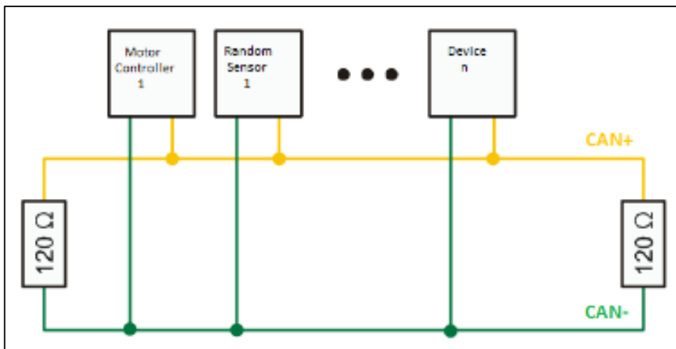
Obrázek 16: Topologie CAN sběrnice se zakončovacími odpory
