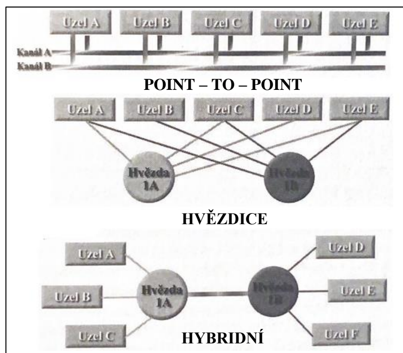
Obrázek 18: Možnosti zapojení FlexRay sběrnice
