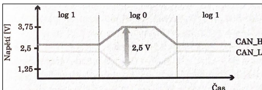
Obrázek 15: Průběh signálu CAN protokolu
