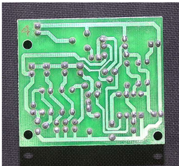
Obrázek 3.3 Testovací deska – spodní strana
