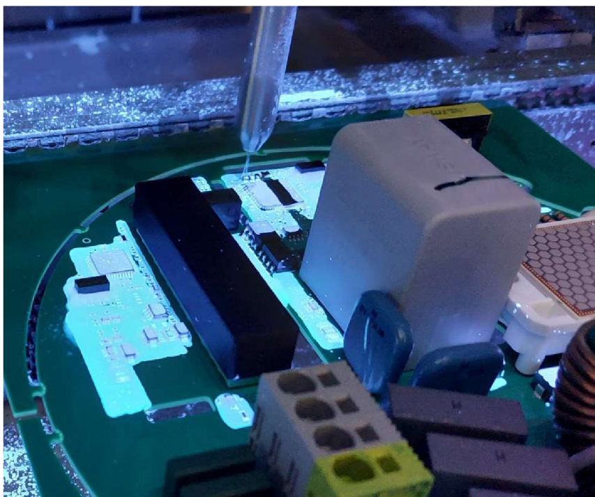
Obrázek 1.2 Nanášení laku sprejem
