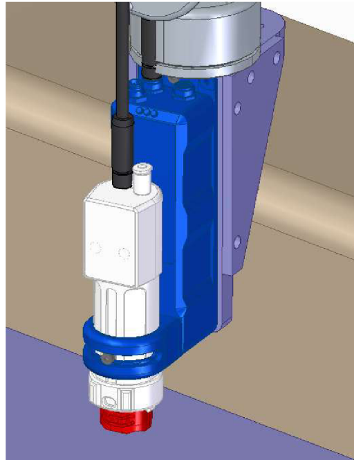
Obrázek 3.26 Detail uchycení vyvíječe plazmy
