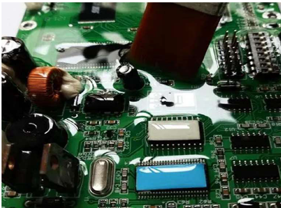
Obrázek 1.4 Silikonový povlak
