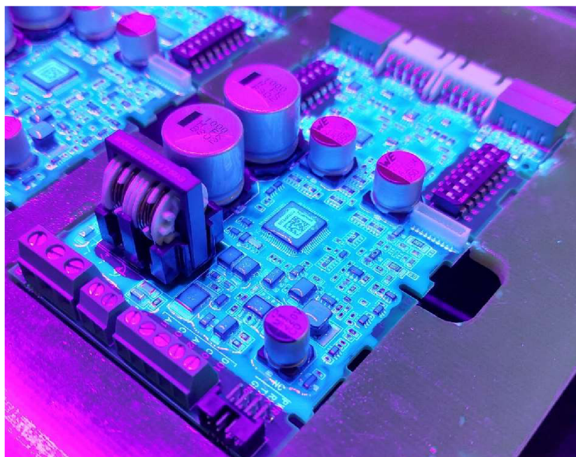
Obrázek 1.1 Konformní povlak
