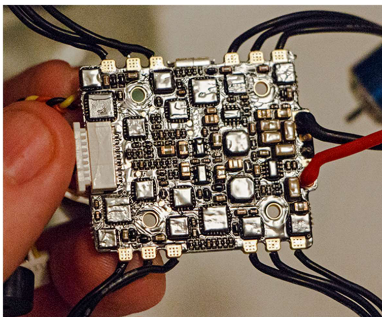
Obrázek 1.3 Akrylový povlak
