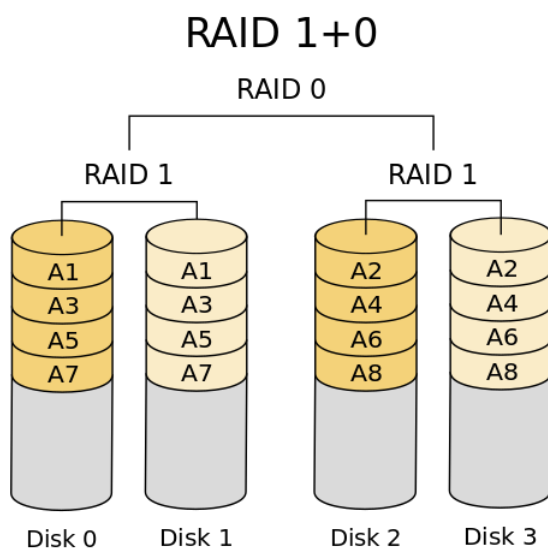
Obrázek 12 RAID 1+0
