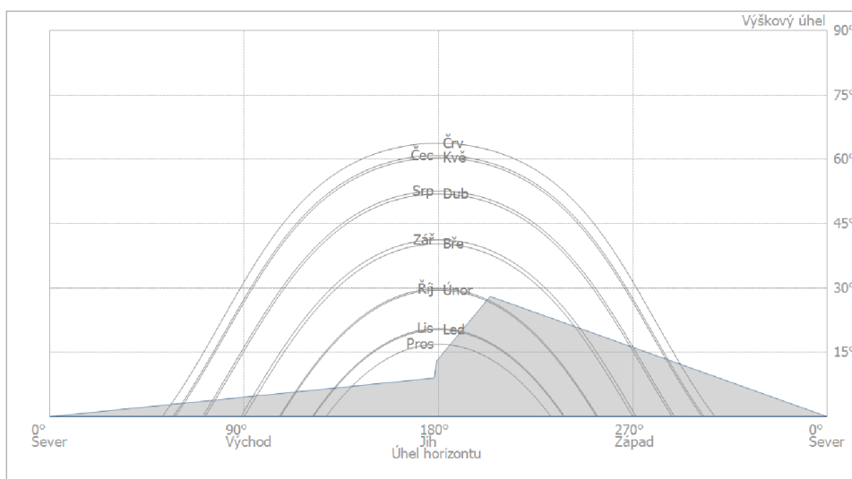
Obrázek: Horizont (3D Návrh)
