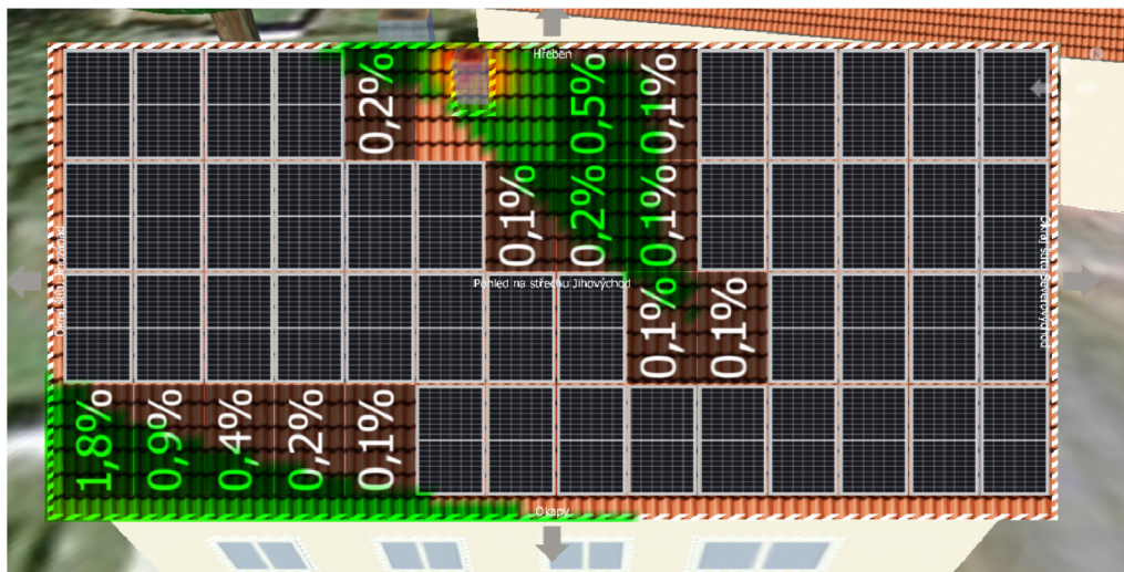
Obr. 2.5: Zastínění panelů rodinného domu.
