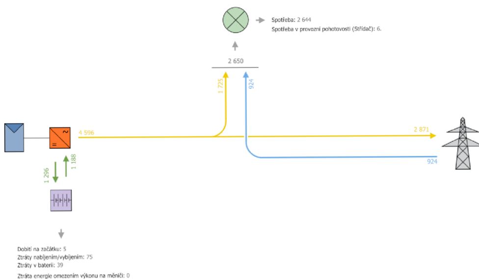
Obr. 2.23: Graf toku energie 4,9kW.
