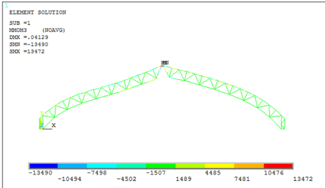
Obr. 5.6 Ohybové momenty na vazníku s průběžnými pásy a kloubově připojenými svislicemi a diagonálami – M3 (K3)
