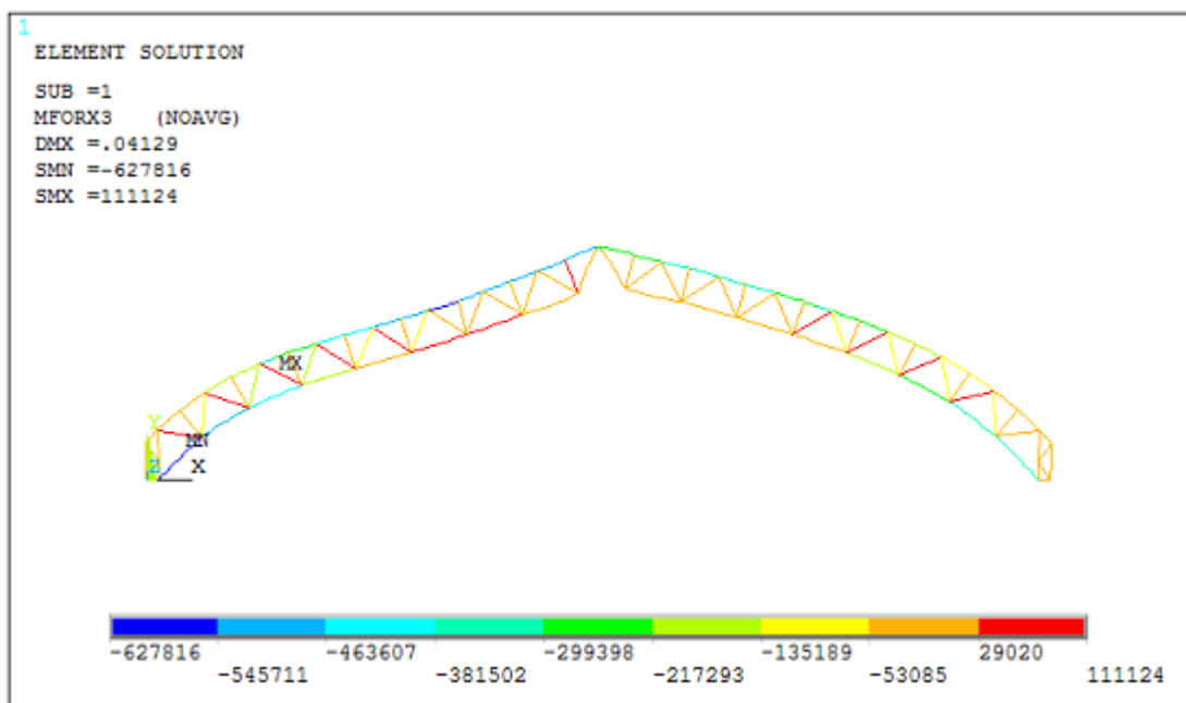
Obr. 5.5 Normálové síly na vazníku s průběžnými pásy a kloubově připojenými svislicemi a diagonálami – M3 (K3)
