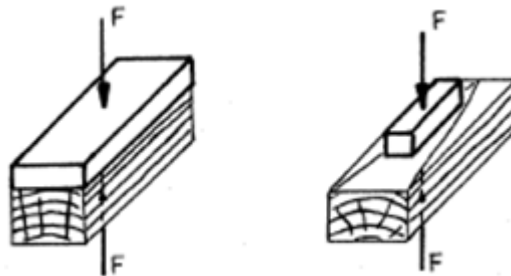
Obr. 3.4 Tlak kolmo na vlákna v radiálním směru
