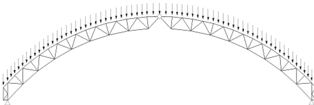
Obr. 4.8 Schéma vazníku s tuze připojenými pruty
