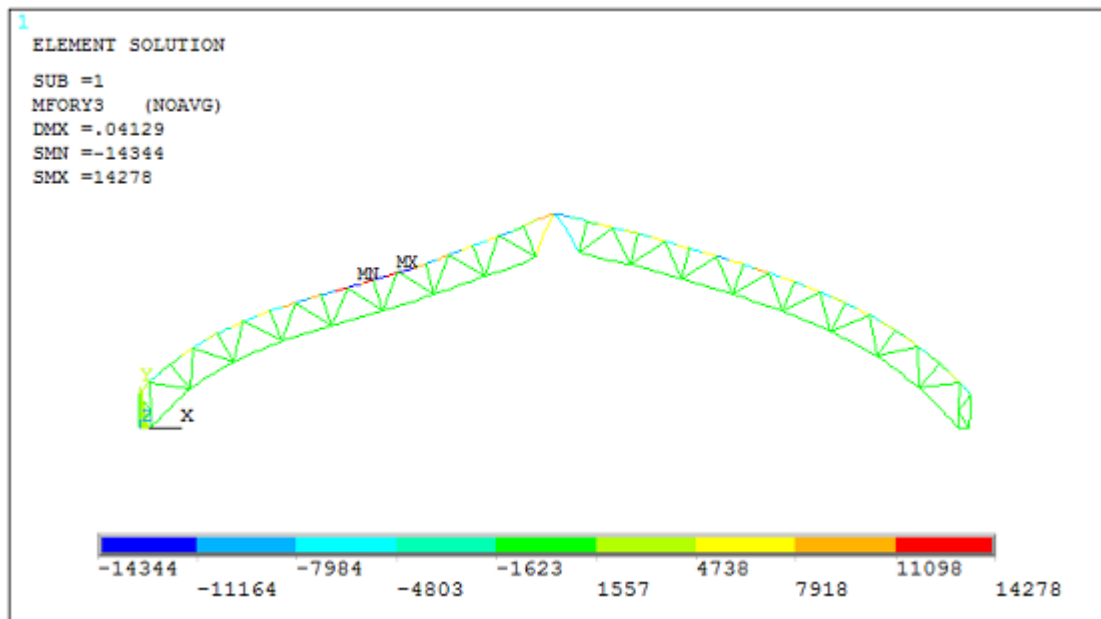
Obr. 5.7 Posouvající síly na vazníku s průběžnými pásy a kloubově připojenými svislicemi a diagonálami – M3 (K3)
