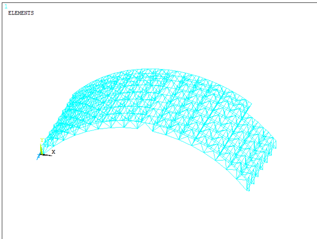
Obr. 4.10 3D model s tuze připojenými prvky
