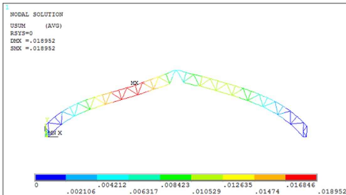
Obr. 5.13 Průhyb ve čtvrtině vazníku s průběžnými pásy a kloubově připojenými svislicemi a diagonálami – M3 (K8)
