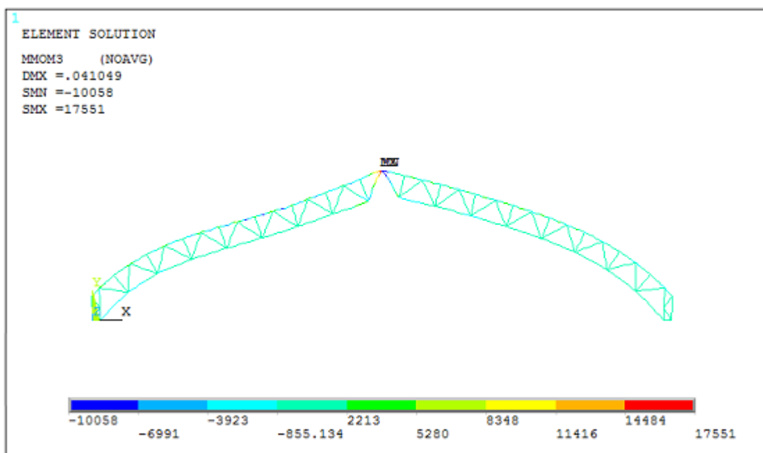
Obr. 5.3 Ohybové momenty na vazníku s tuze připojenými pruty – M2 (K3)
