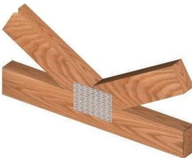
Obr. 2.5 Deska s prolisovanými trny [37]
