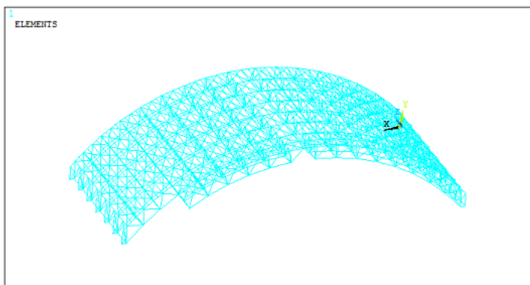
Obr. 4.11 3D model s tuze připojenými prvky
