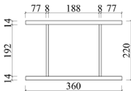
Obr. 4.15 Použité průřezy vazníku
