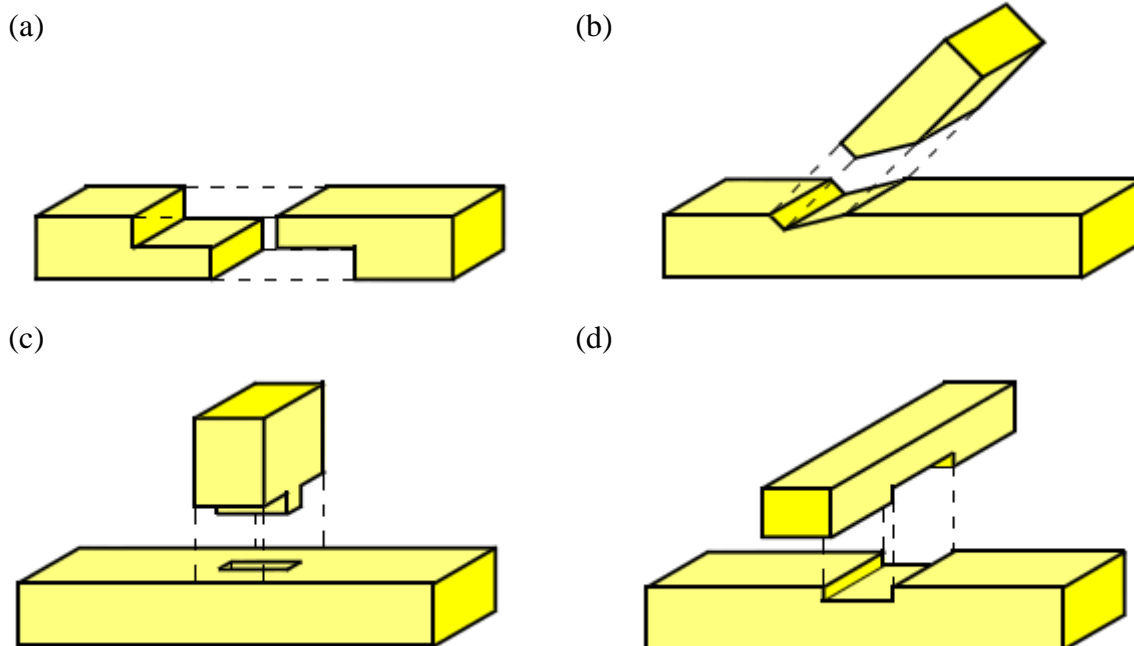
Obr. 2.3 Základní typy tesařských spojů: (a) přeplátování, (b) zapuštění, (c) čepování, (d) karpování [13]
