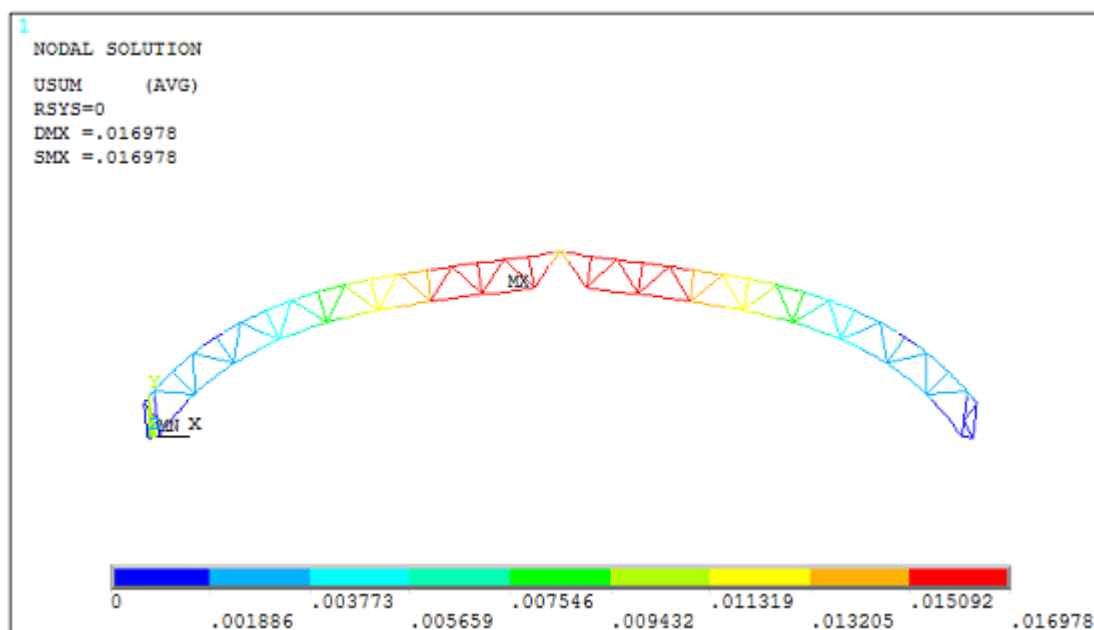
Obr. 5.12 Průhyb ve vrcholu vazníku s průběžnými pásy a kloubově připojenými svislicemi a diagonálami – M3 (K6)
