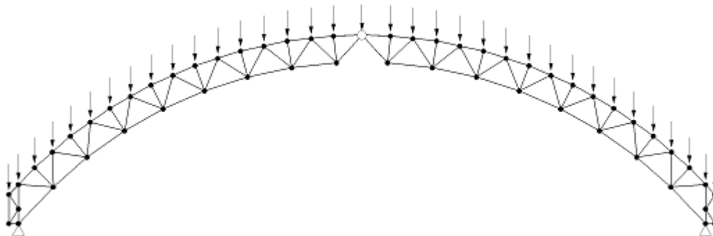
Obr. 4.7 Schéma vazníku s kloubově připojenými pruty
