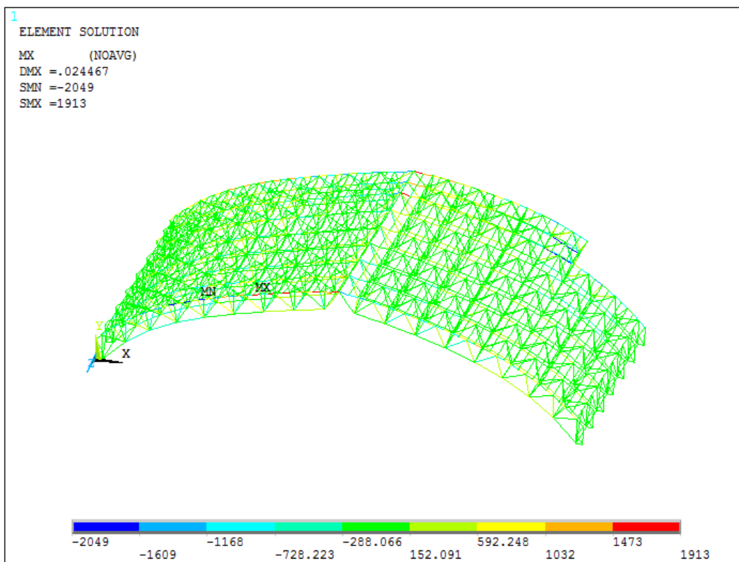
Obr. 5.18 Kroutící moment M_x 3D modelu s tuze připojenými pruty (K3)
