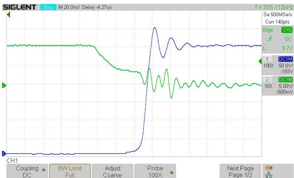
Obrázok 25 Detail vypínacieho deja výkonového tranzistora
