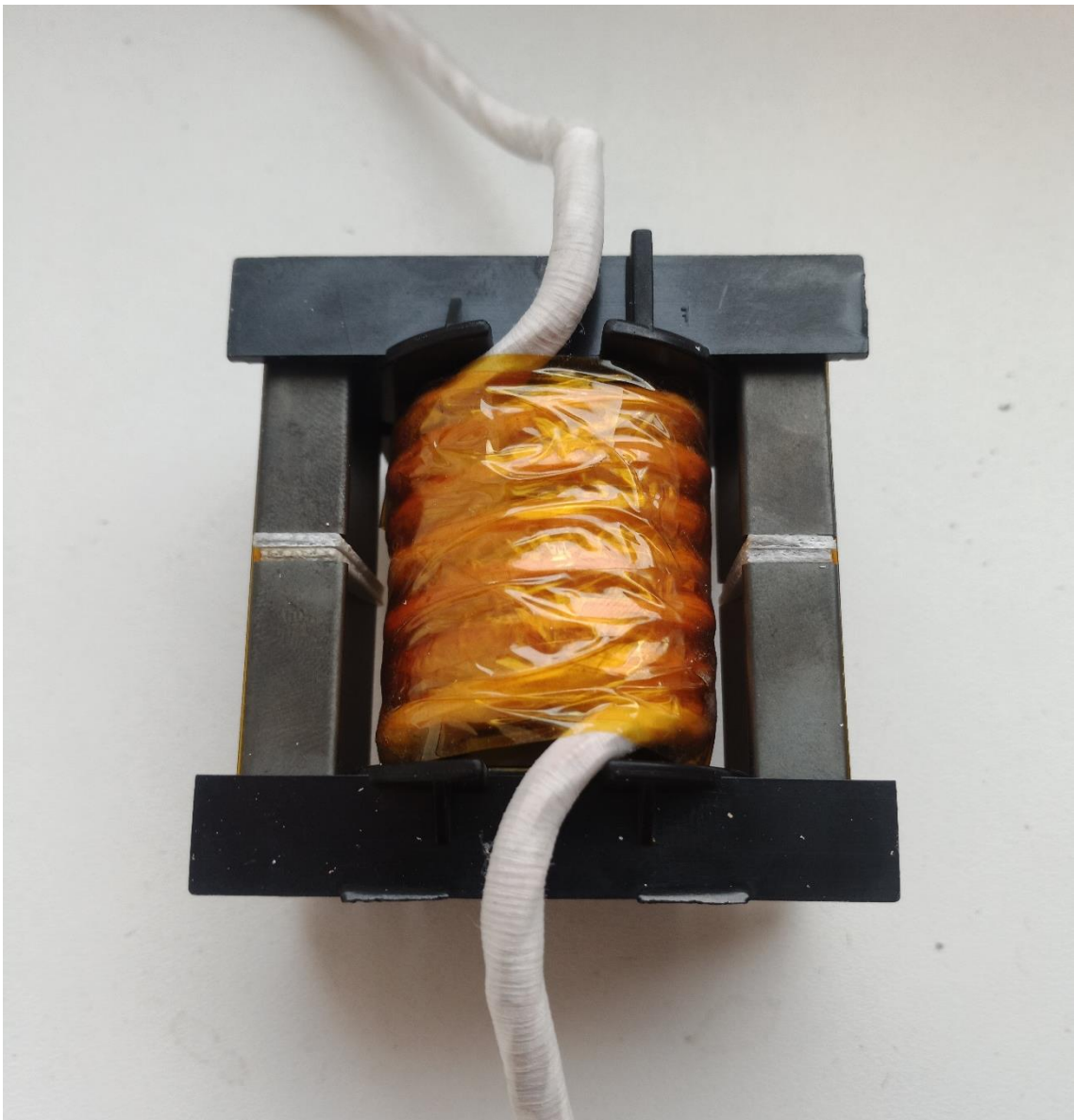
Obrázok 11 Výstupná tlmivka
