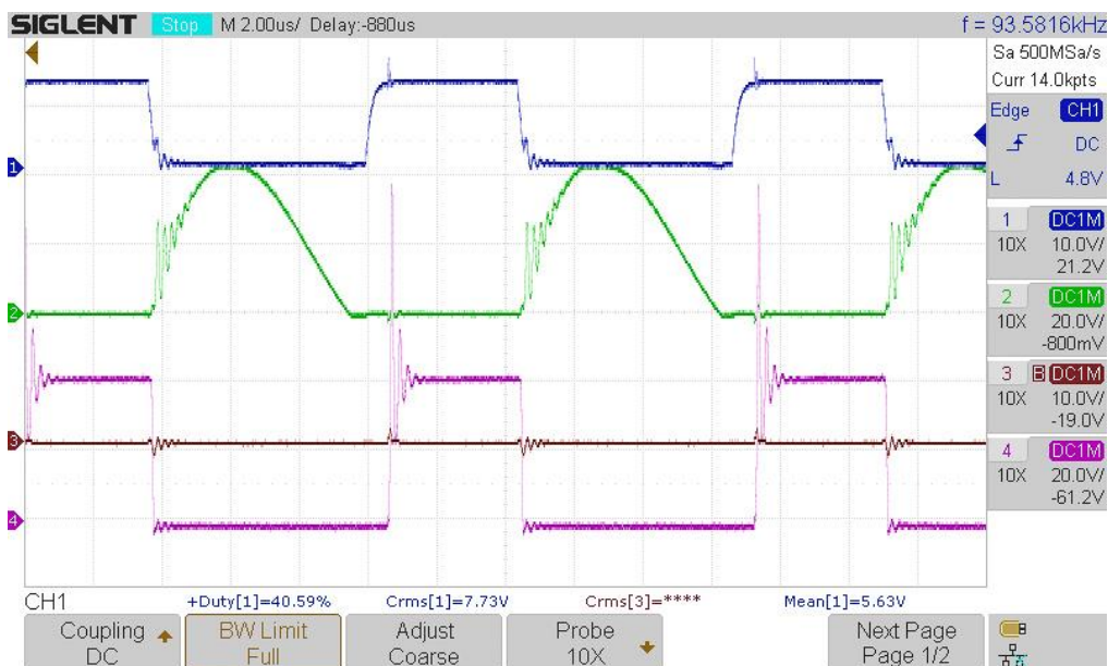
Obrázok 30 Priebehy napätí synchronného usmerňovača pri prúde 9,2 A
