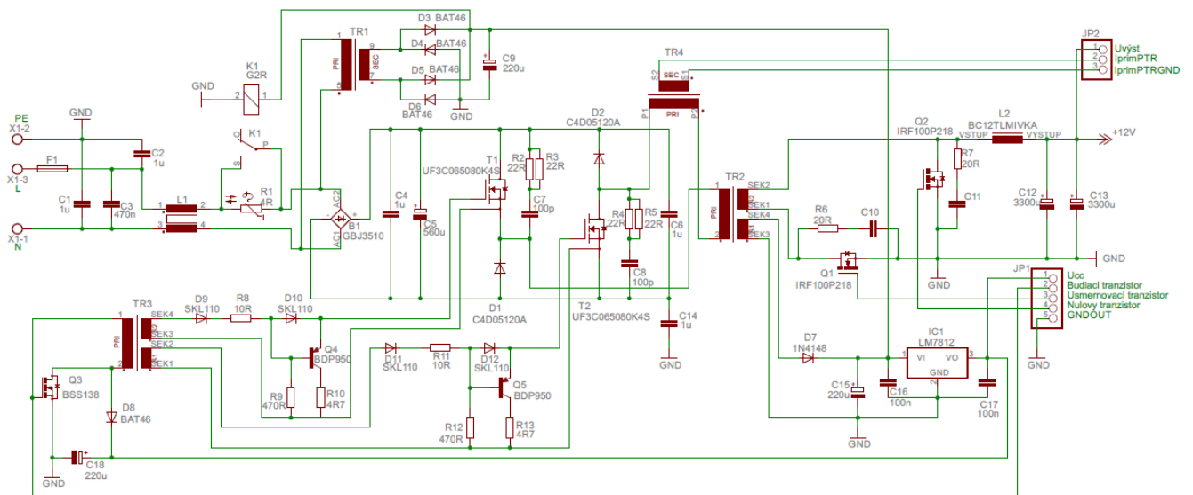
Obrázok 5 Výsledná schéma silového obvodu
