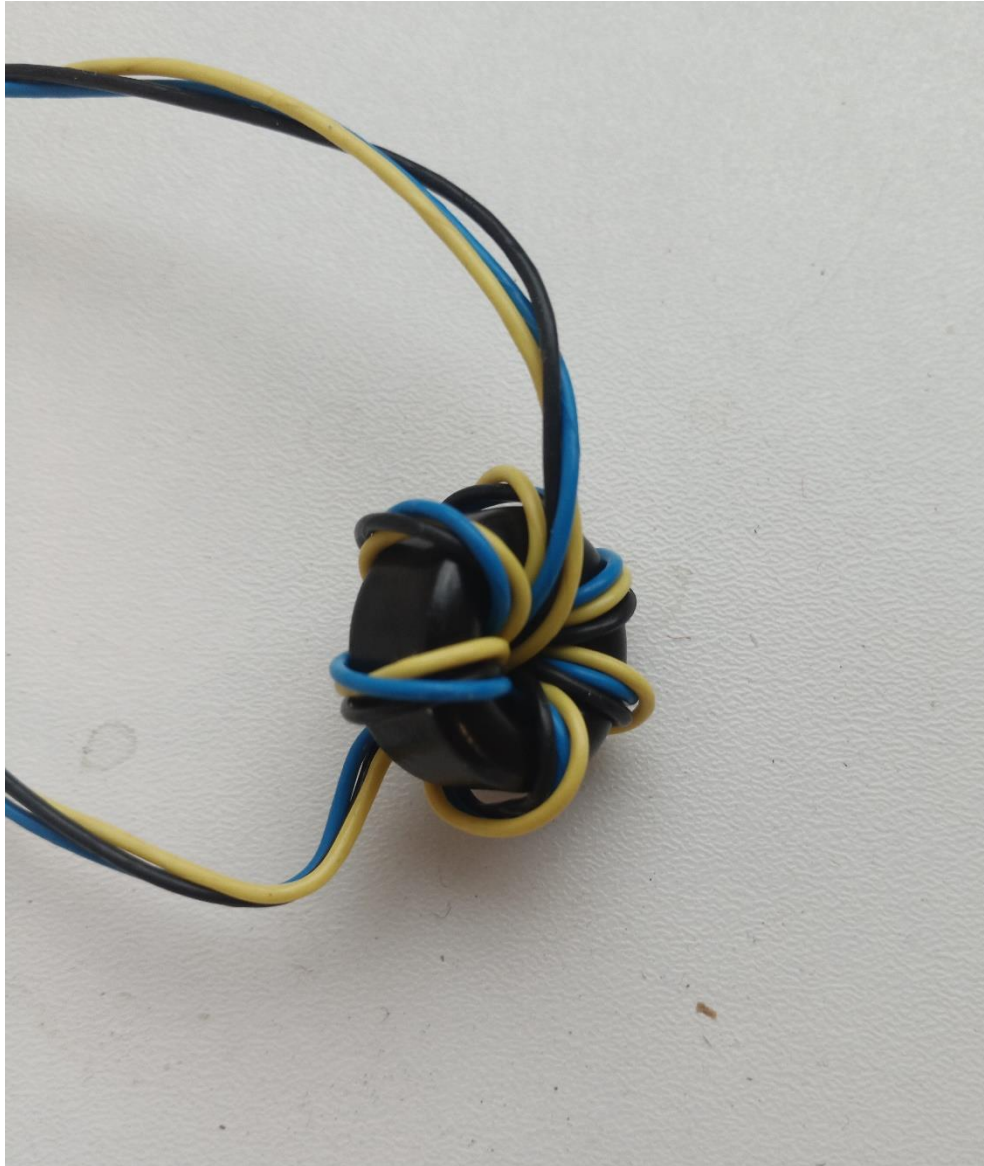
Obrázok 13 Budiaci transformátor
