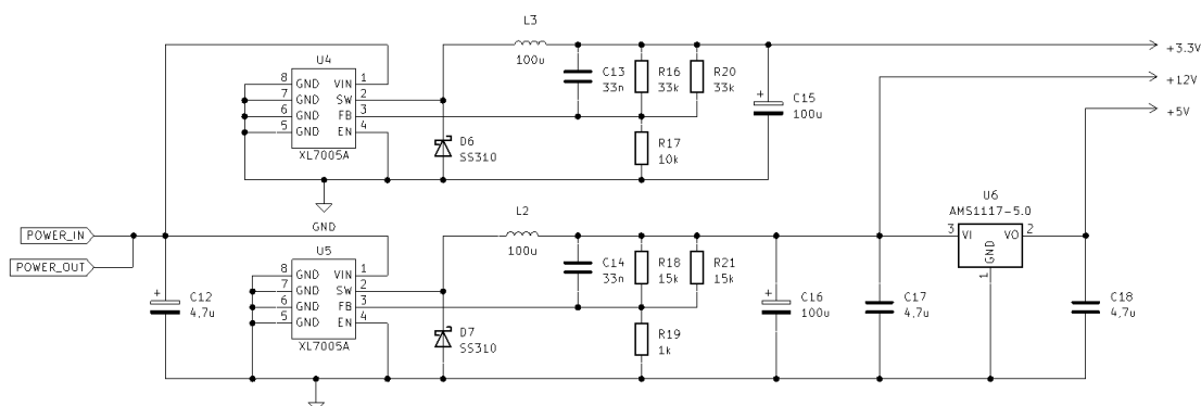
Obrázek 10-5 Schéma napájecí části MPPT
