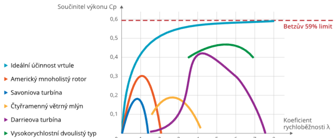
Obrázek 2-5 Závislost součinitele výkonosti na koeficientu rychloběžnosti pro vybrané větrné turbíny [7]
