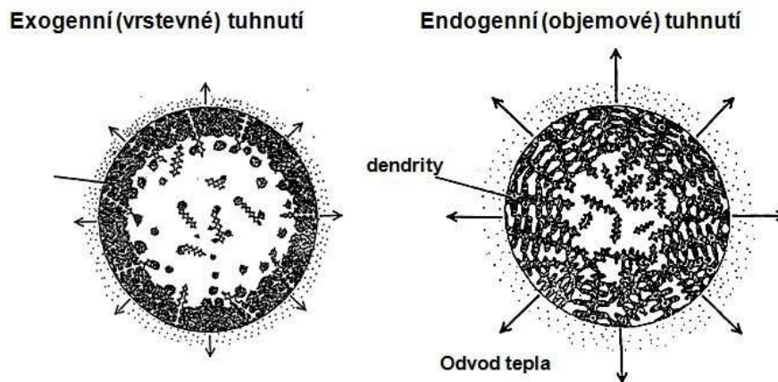
Obr. 13 Exogenní a endogenní tuhnutí [18]
