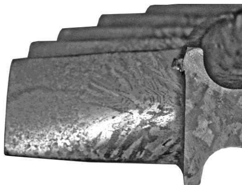
Obr. 72 Lopatka kola č. 62
