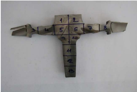
Obr. 29 Rozdělení metalografických vzorků
