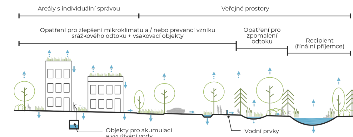
OBR. Č. 40 SCHÉMA DEŠŤOVÉHO ŘETĚZCE, zdroj: Sýkorová et al. 2022, str. 36
