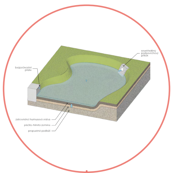
VSAKOVACÍ RETENČNÍ NÁDRŽ
