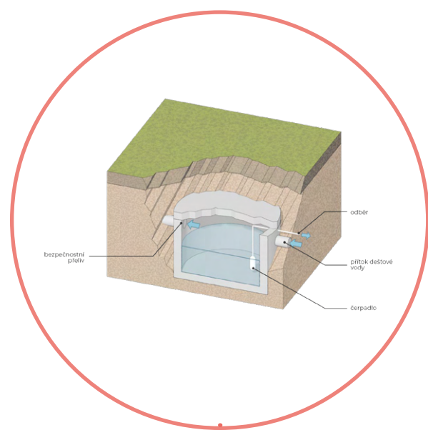
POZDEMŇNÍ RETENČNÍ DEŠŤOVÁ NÁDRŽ
