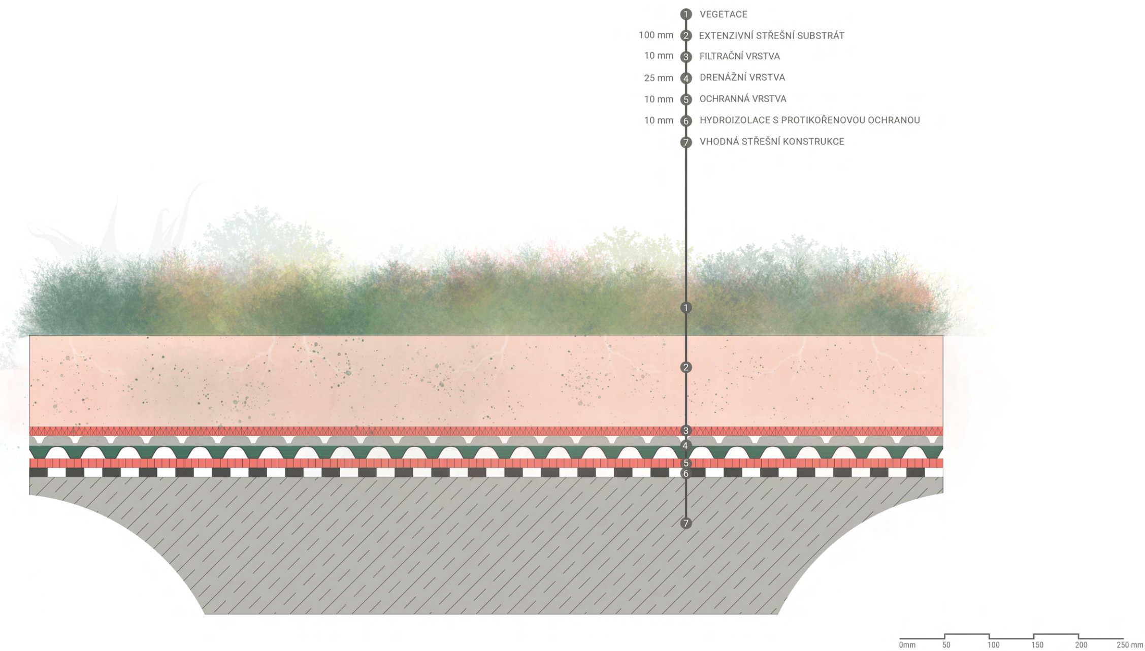
OBR. Č. 118 SOUVRSTVÍ EXTENZIVNÍ STŘECHY, zdroj: optigruen.de + autor práce
