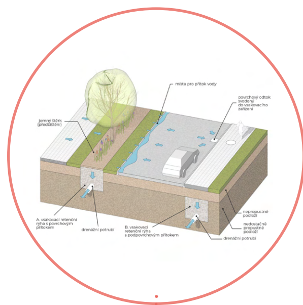
VSAKOVACÍ RETENČNÍ RÝHA A JEJÍ VARIANTY
