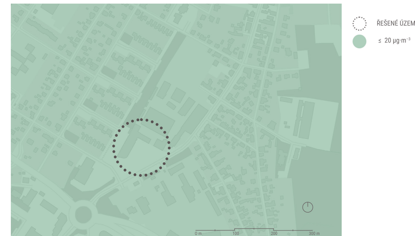
OBR. Č. 62 KONCENTRACE PEVNÝCH ČÁSTIC PM 10 , zdroj: geoportalpraha.cz + chmi.cz + autor práce
