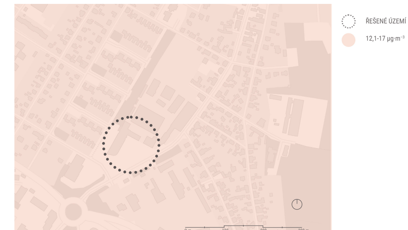
OBR. Č. 63 KONCENTRACE PEVNÝCH ČÁSTIC PM 2,5 , zdroj: geoportalpraha.cz + chmi.cz + autor práce
