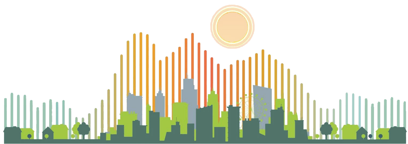
OBR. Č. 4 EFEKT TEPELNÉHO OSTROVA, zdroj: buildpass.co.uk
