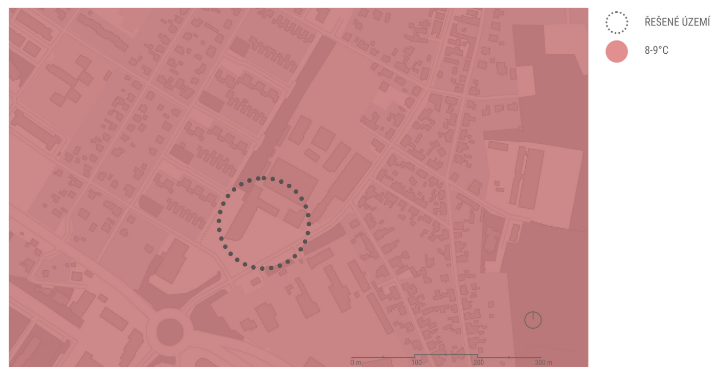
OBR. Č. 60 PRŮMĚRNÁ ROČNÍ TEPLOTA, zdroj: geoportalpraha.cz + chmi.cz + autor práce
