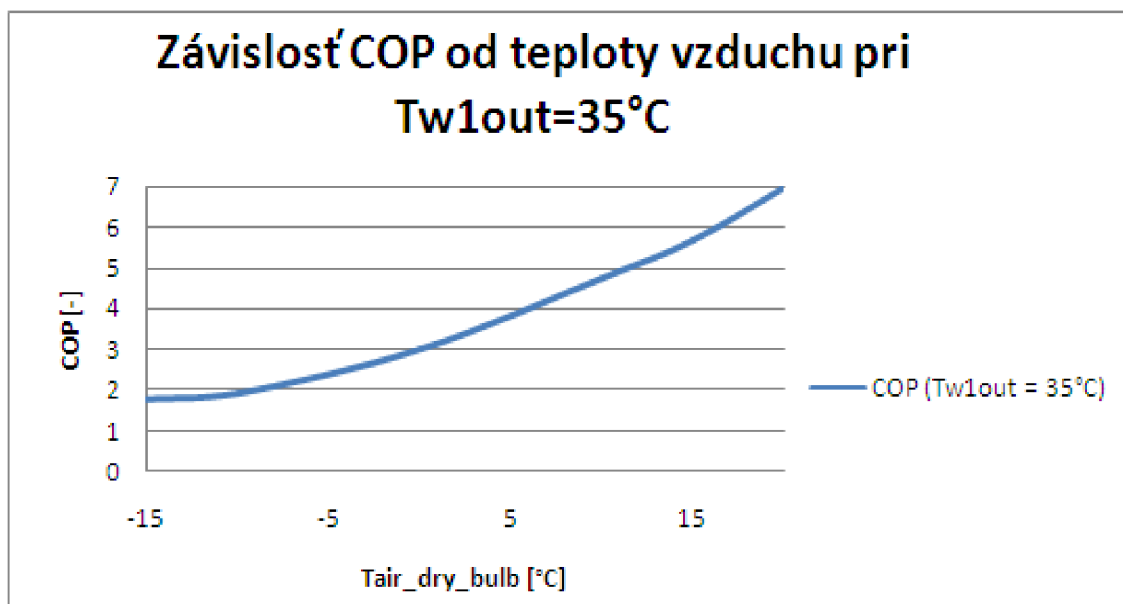
Obr. 9.3 Závislosť výkonového čísla COP od teploty vzduchu T_{w1out}=35^{\circ}\text{C}
