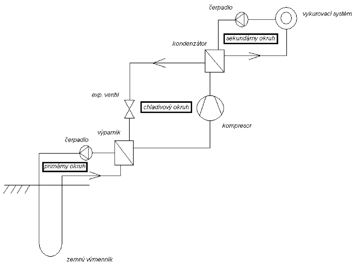
Obr. 1.1 Okruhy TČ
