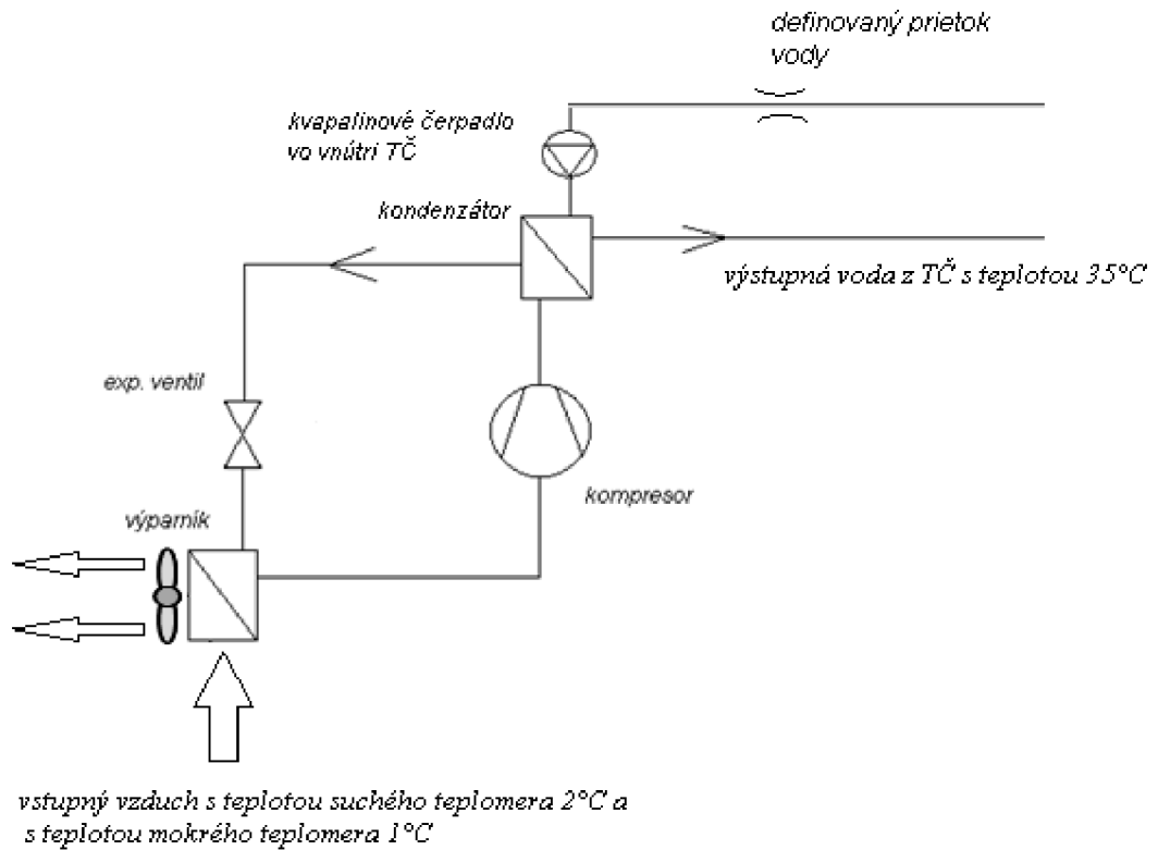
Obr. 1.2 Konštantné podmienky
