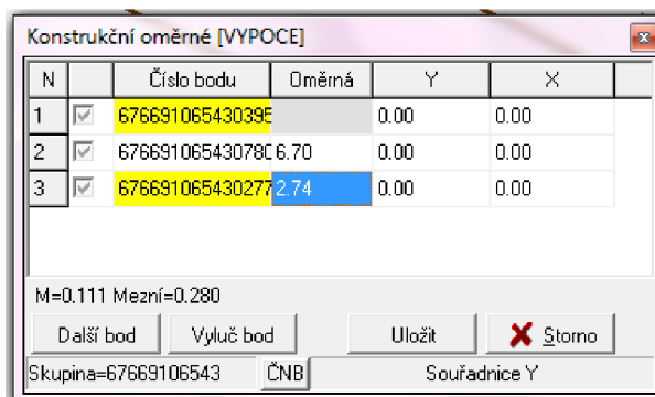
Obr. 13 Konstrukční oměrné
