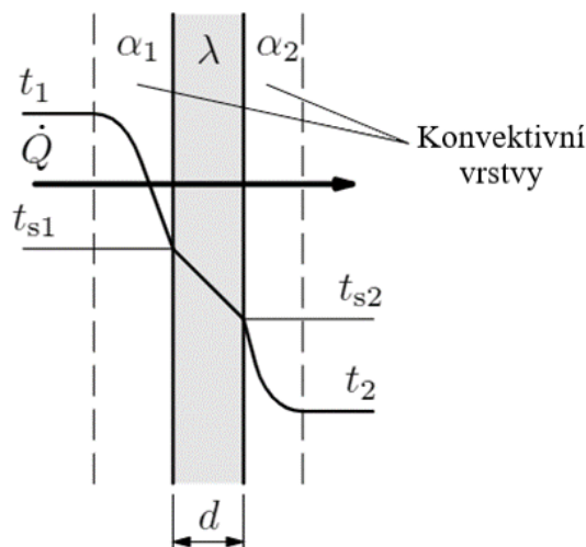
Obrázek 3.4 Vedení a prostup tepla rovinnou stěnou [51].
