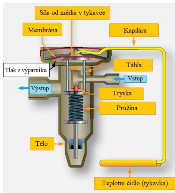
Obrázek 1.9 Expanzní ventil s vnitřním vyrovnáním tlaku [28].
