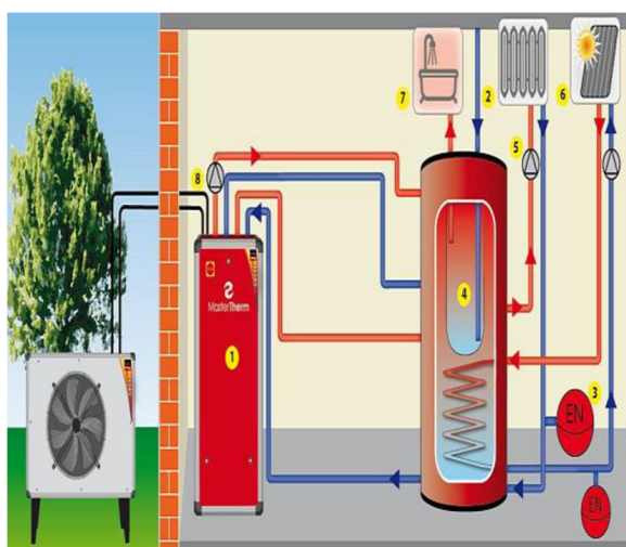
Obrázek 32: tepelné čerpadlo vzduch-voda [57]
