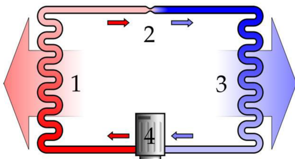
Princip tepelného čerpadla :
