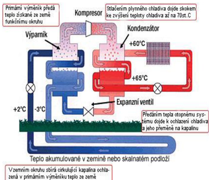
Obrázek 35: tepelné čerpadlo země-voda [60]
