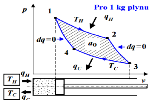
Obrázek 27: Cartonův cyklus [49]
