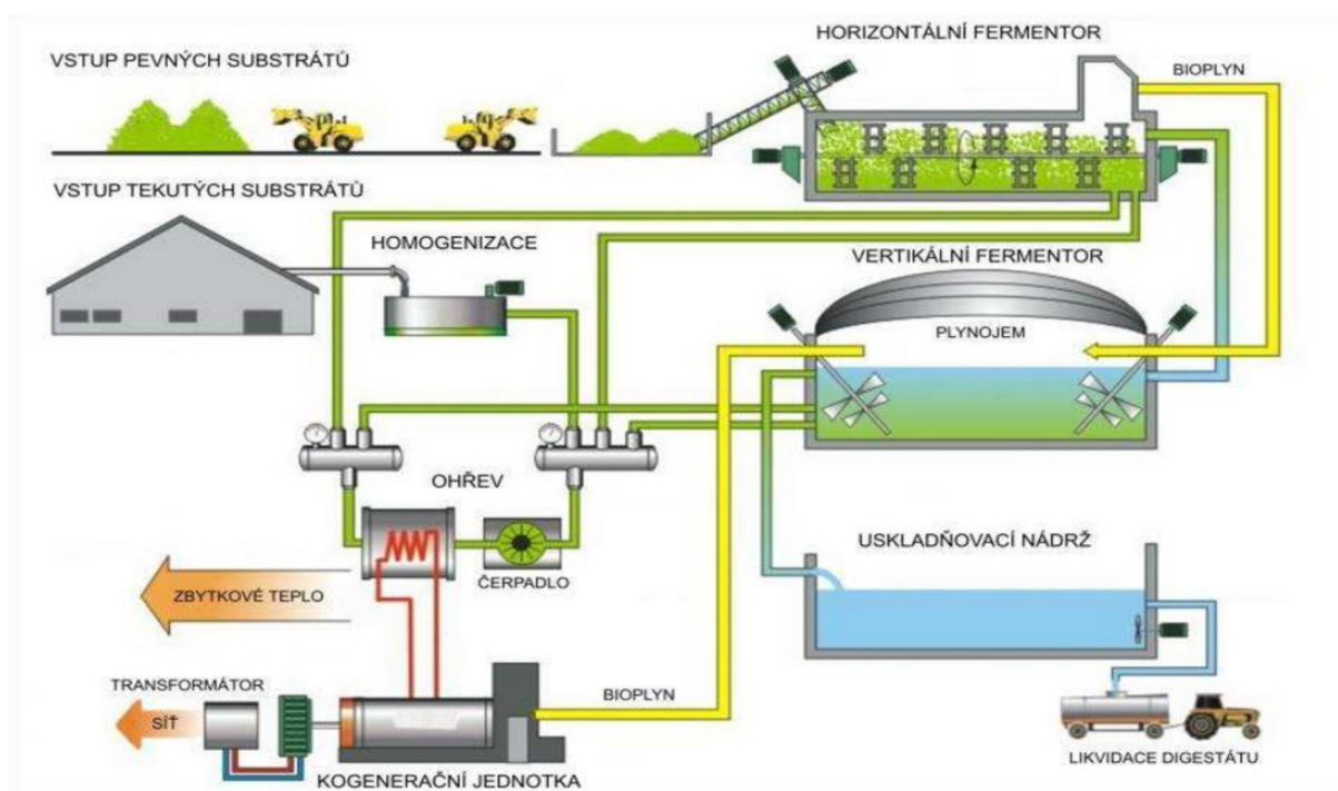
Obrázek 18: Bioplynová stanice [34]
