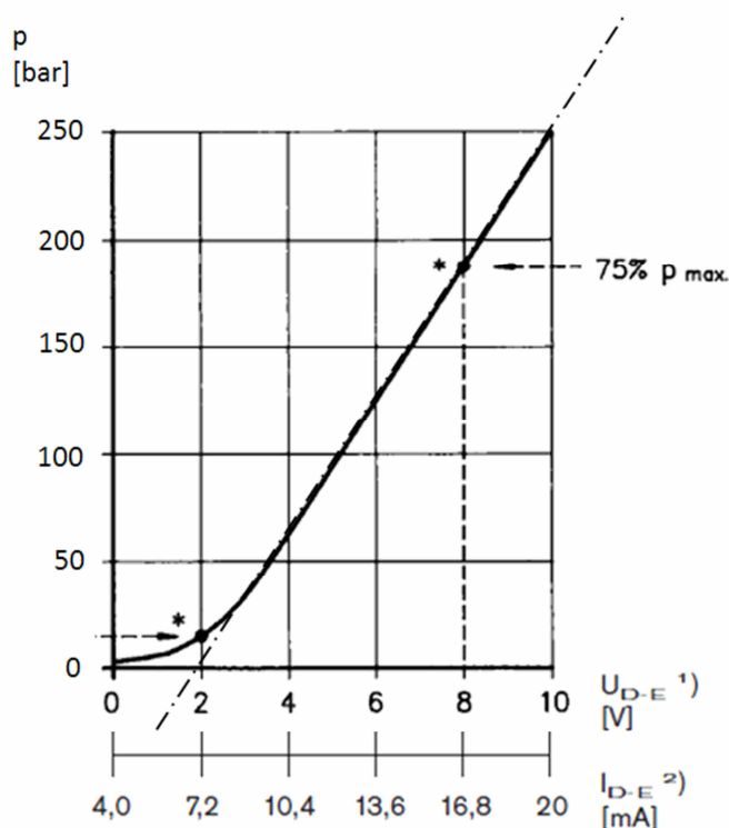
Obr.14 Závislost tlaku na řídicím signálu proporcionálního tlakového ventilu s elektronickou zpětnou vazbou [10]
