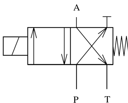
Obr.13 Schématická značka čtyřcestného dvoupolohového rozvaděče.
