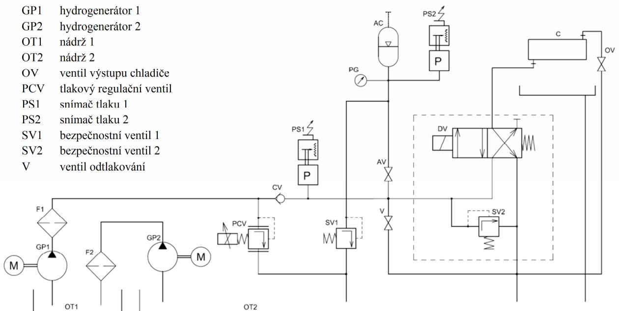
Obr.36 Hydraulické schéma
