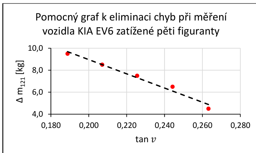
Graf 57 Pomocný graf k eliminaci chyb při měření vozidla KIA EV6 zatíženého pěti figuranty
