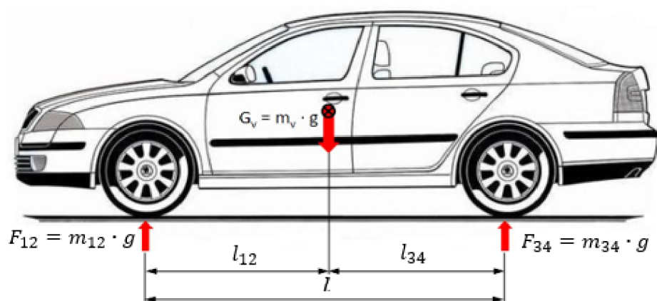
Obr. 4 Měření podélné polohy těžiště vozidla [2]
