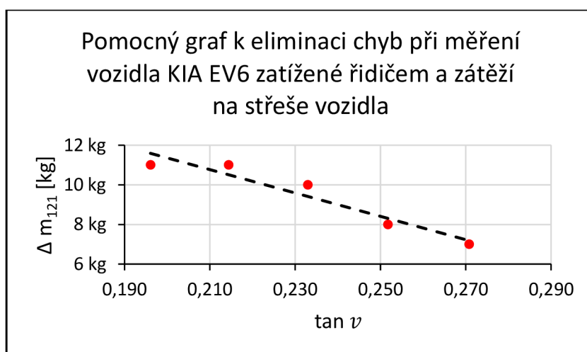
Graf 58 Pomocný graf k eliminaci chyb při měření vozidla KIA EV6 zatíženého řidičem a zátěží na střeše vozidla
