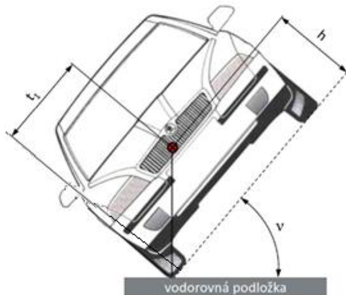
Obr. 8 Metoda zjištění úhlu překlpení [2]
