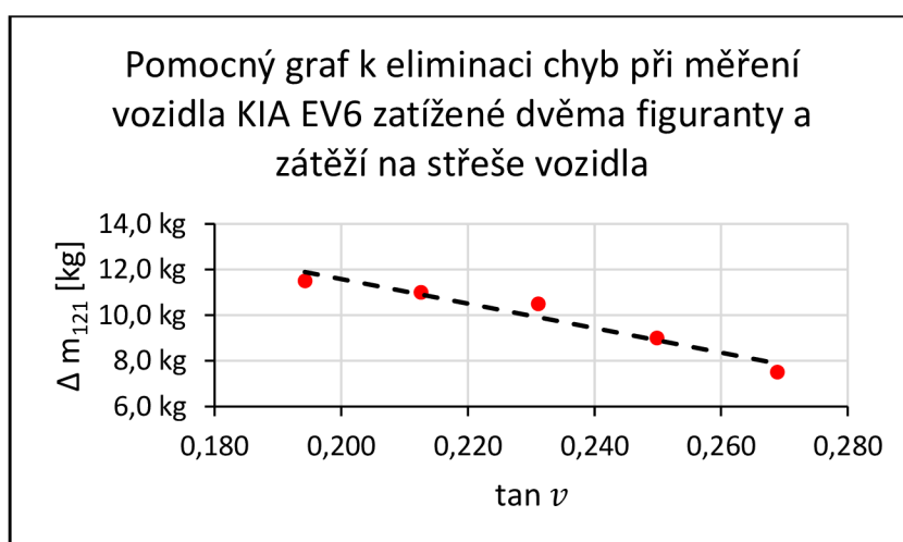
Graf 59 Pomocný graf k eliminaci chyb při měření vozidla KIA EV6 zatíženého dvěma figuranty a zátěží na střeše vozidla
