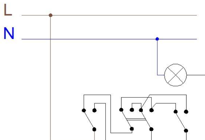
Obr. 6-7 Zapojení pro ovládání z více jak dvou míst (Upraveno podle [6])
