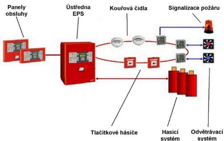
Obr. 5-6 Příklad požárního systému (Upraveno podle [9]).
