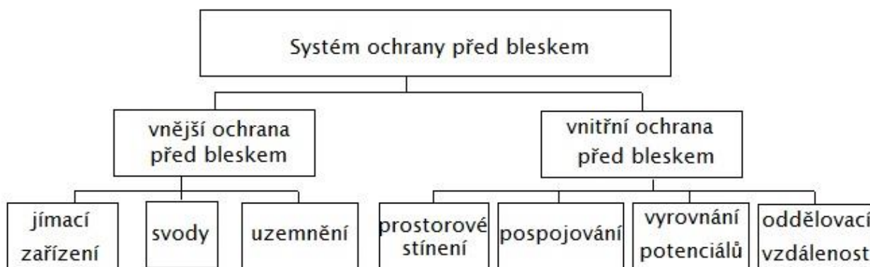
Obr. 7-1 Rozdělení systému ochrany před bleskem (Upraveno podle [5]).
