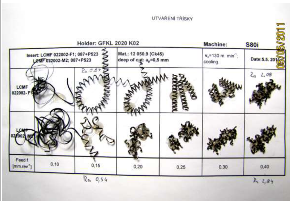
Obrázek 4.1 Tváření třísek při podélném soustružení v hloubce záběru a_p = 0,5 mm 4
