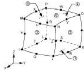
Obr. 6.3 Použitý prvek SOLID90
