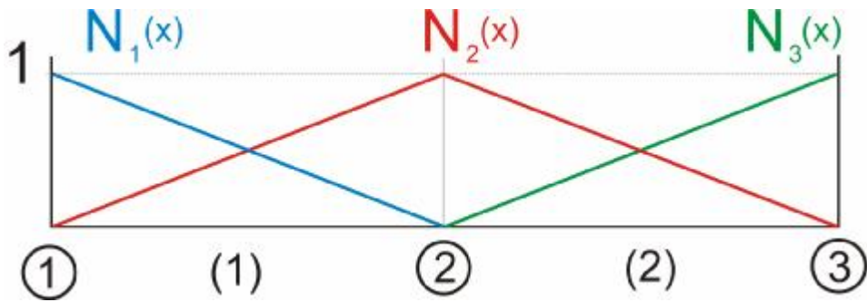
Obr. 1.3 Bázové funkce
