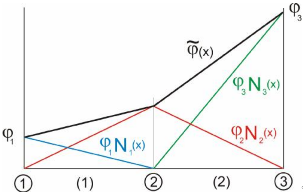
Obr. 1.4 Globální aproximace
