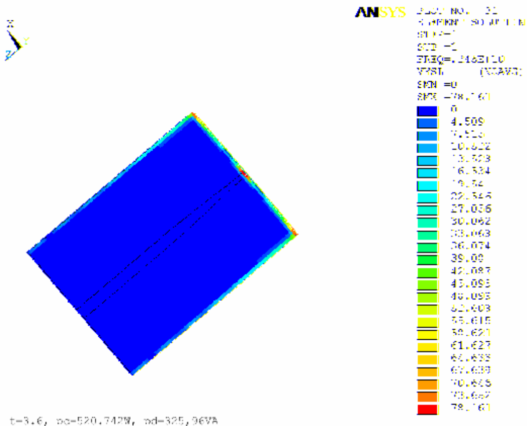
Obr. 8.4 Rozložení činných ztrát v emulzi pro t=3,6 s
