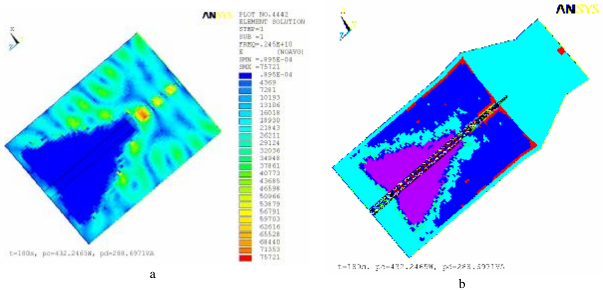
Obr. 8.9 a) Rozložení intenzity elektrického pole v emulzi, b) vysušené elementy, t=180 s
