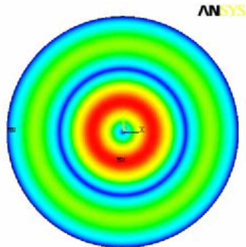
Obr. 5.3 Příčné rozložení E pro vid TE_{02}
