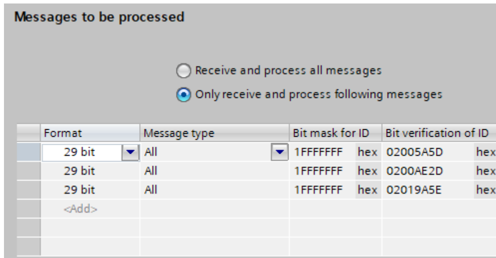
Obrázek 7 – Nastavení filtru přijatých zpráv uvnitř HSP
