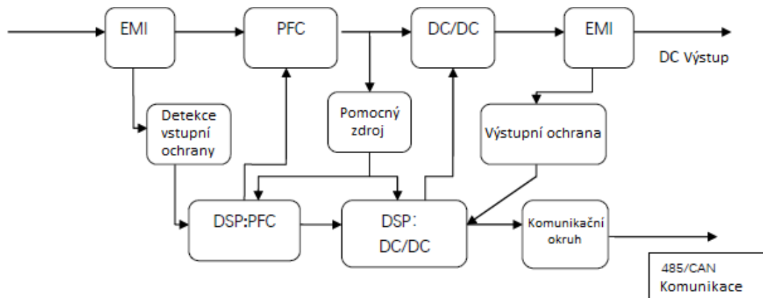
Obrázek 2 - Princip funkce modulu UR50060-E [5]
