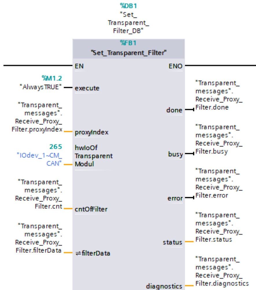
Obrázek 16 – Funkční blok pro nastavení filtrů přijímaných CAN zpráv
