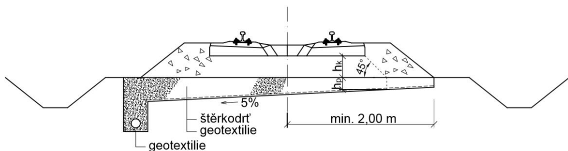
Obr. 5.4 PŘÍČNÝ ŘEZ KONSTRUKCE S POUŽITOU GEOTEXTILÍ A ODVODNĚNÍM DO TRATIVODU [1]
