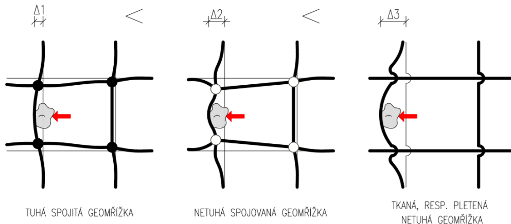
Obr. 5.11 VLIV TUHOSTI GEOMŘÍŽKY NA STABILITU OKA PŘI ZATÍŽENÍ
