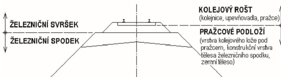
Obr. 2.1 DĚLENÍ ŽELEZNIČNÍHO TĚLESA [1]
