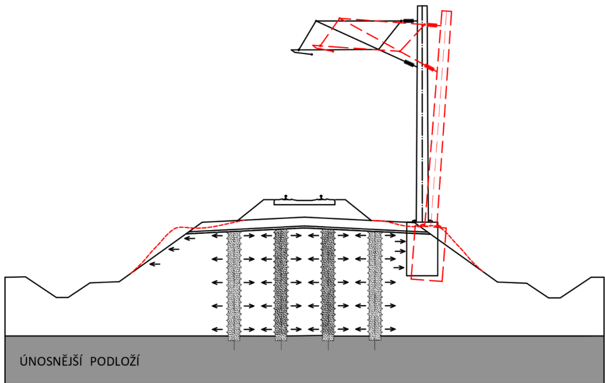
Obr. 6.11 PORUŠENÍ NÁSPU
