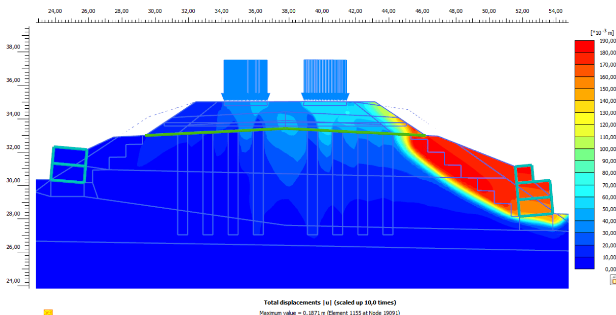
Obr. 7.10 FÁZE 12: POLOHA KRITICKÉ SMYKOVÉ PLOCHY (STABILITA SANOVANÉHO TĚLESA ZATÍŽENÉHO DOPRAVOU 80kN/m, IZOPLOCHY CELKOVÝCH POSUNŮ)
