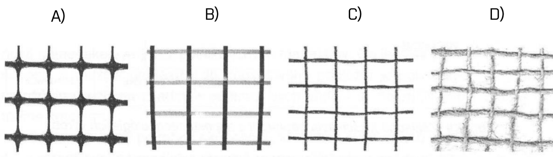
Obr. 5.8 DĚLENÍ DLE TUHOSTI GEOMŘÍŽKY [19]
