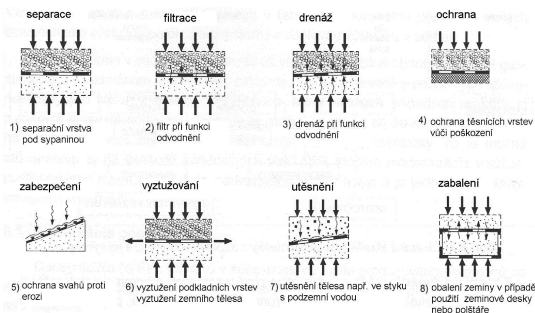
Obr. 5.1 FUNKCE GEOSYNTETIK [19]
