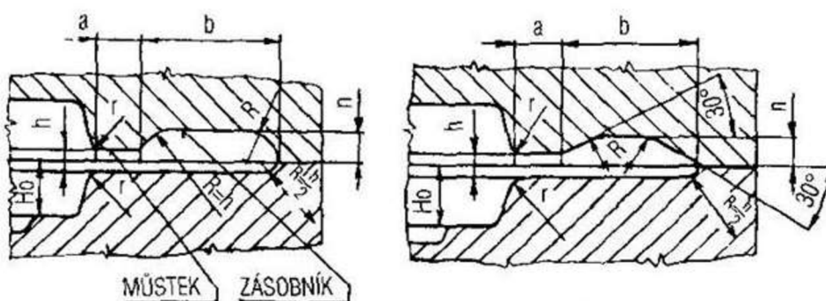
Obr. 24 Výronkové drážky zápusťek pro buchar [23]
