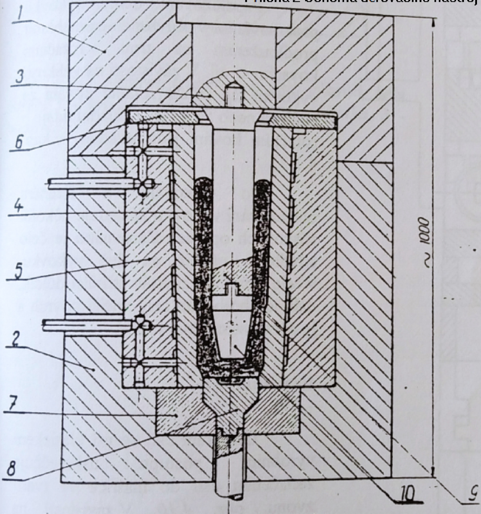
Příloha 2 Schéma děrovacího nástroj
