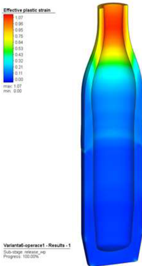
Obr. 48 Finální tvar přivření
