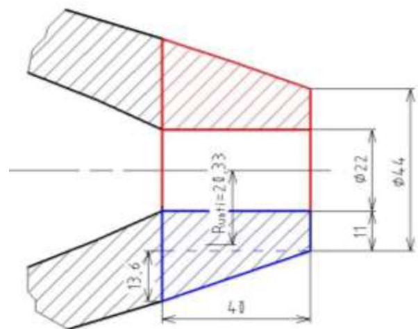
Obr. 38 Řez ústím
