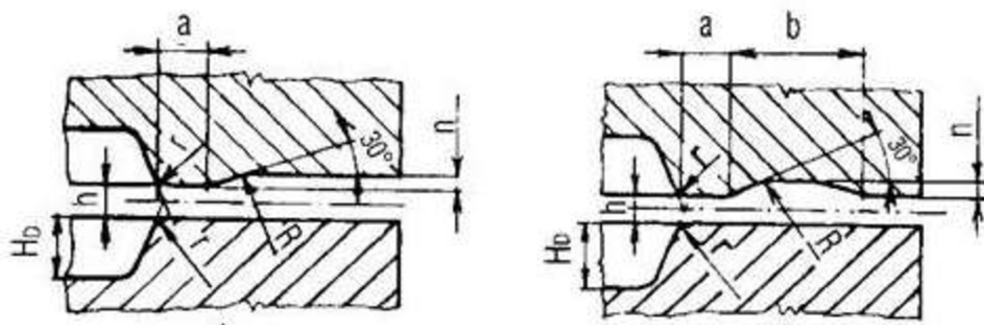
Obr. 26 Výronkové drážky zápustek pro lis [23]
