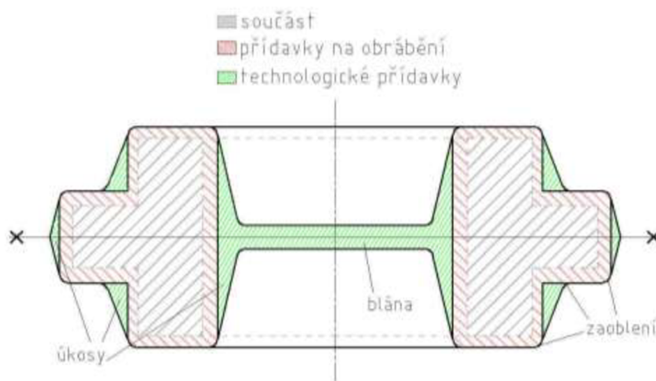
Obr. 22 Přidavky výkovku [20], [32]
