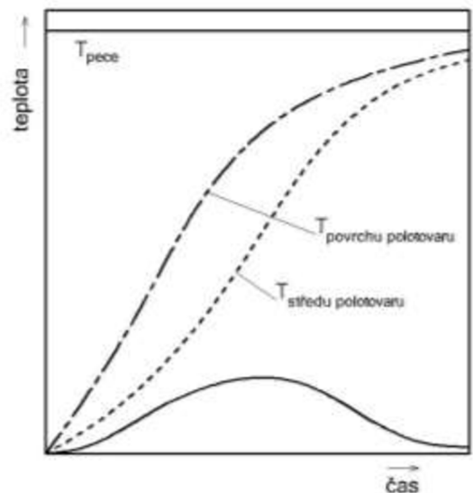
Obr. 15 Režim konstantního ohřevu [16]
