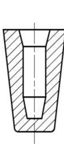
Obr. 33 Děrovaný výkovek
