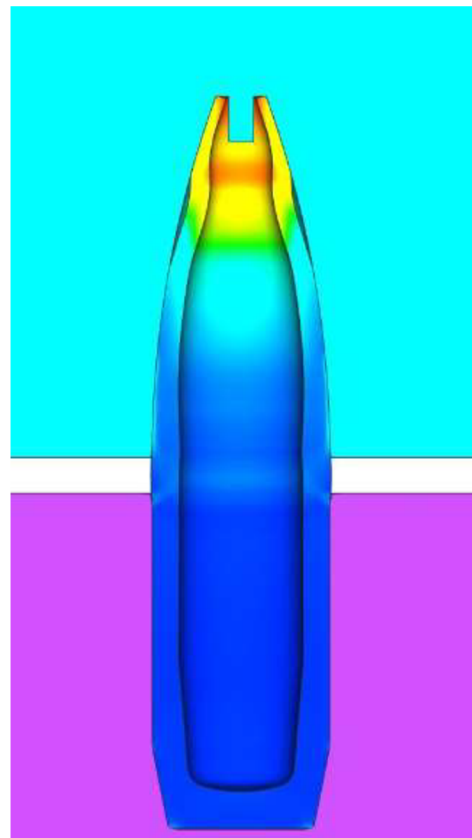
Obr. 49 Pěchování stěny při přídavku 20 mm
