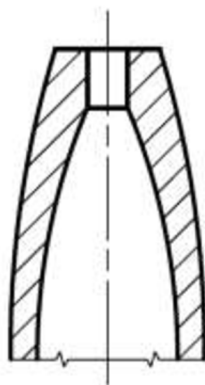
Obr. 37 Uzavřené ústí
