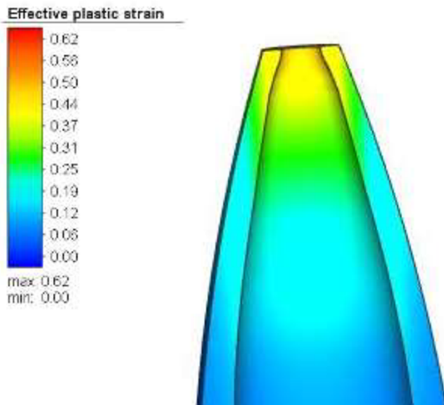
Obr. 50 Výsledek uzavření s přídavkem 15 mm
