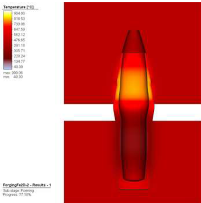
Obr. 41 Okamžik zadření
