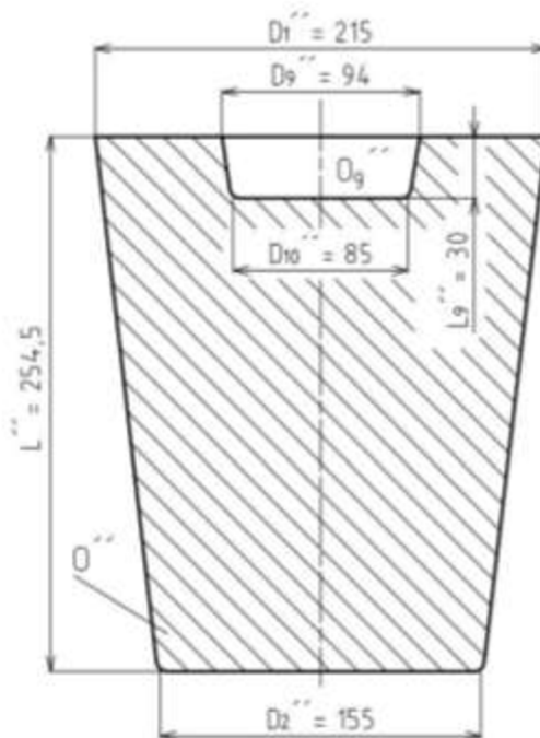
Obr. 57 Předděřovaný výkovek schéma
