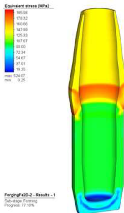
Obr. 42 Vyboulení výkovku
