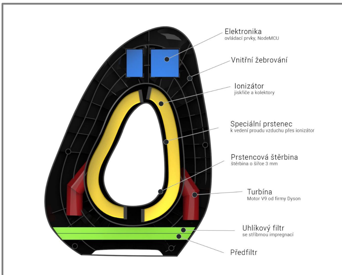
Obr. 5-1 Vnitřní uspořádání navrhované čističky vzduchu
