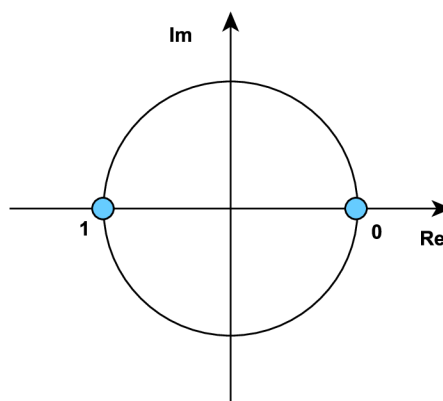
Obr. 3.10: DBPSK
