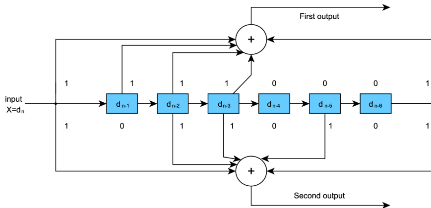
Obr. 3.4: Konvoluční kodér pro omezení K=7 , bitovou rychlost r=1/2
