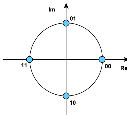
Obr. 3.11: DQPSK
