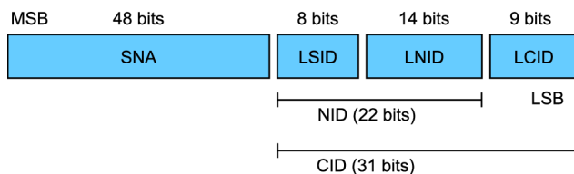
Obr. 3.17: Struktura adresy PRIME
