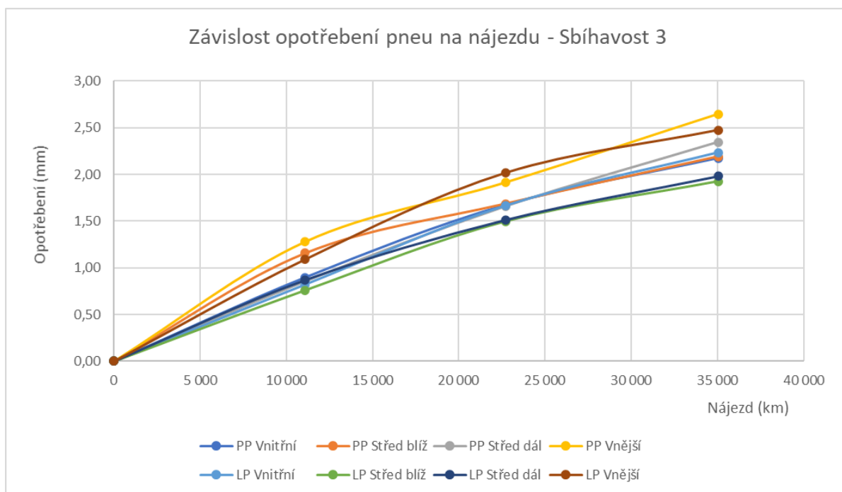
Graf č. 3: Závislost opotřebenění pneumatik na nájezdu – Sbíhavost 3 [vlastní]
