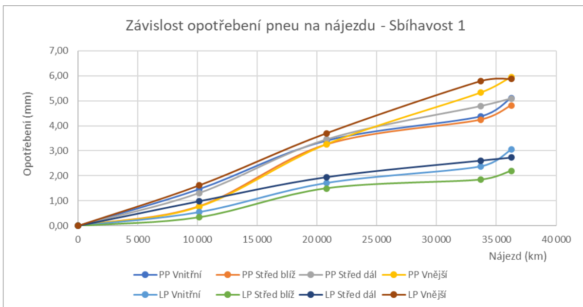
Graf č. 1: Závislost opotřebení pneumatik na nájezdu – Sbíhavost 1 [vlastní]
