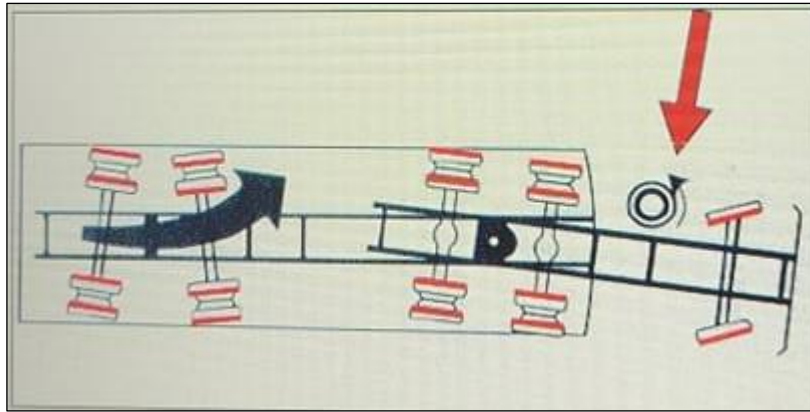
Obr. č. 33: Dvě osy návěsu nejsou umístěny paralelně, volant musí korigovat směr [36]
