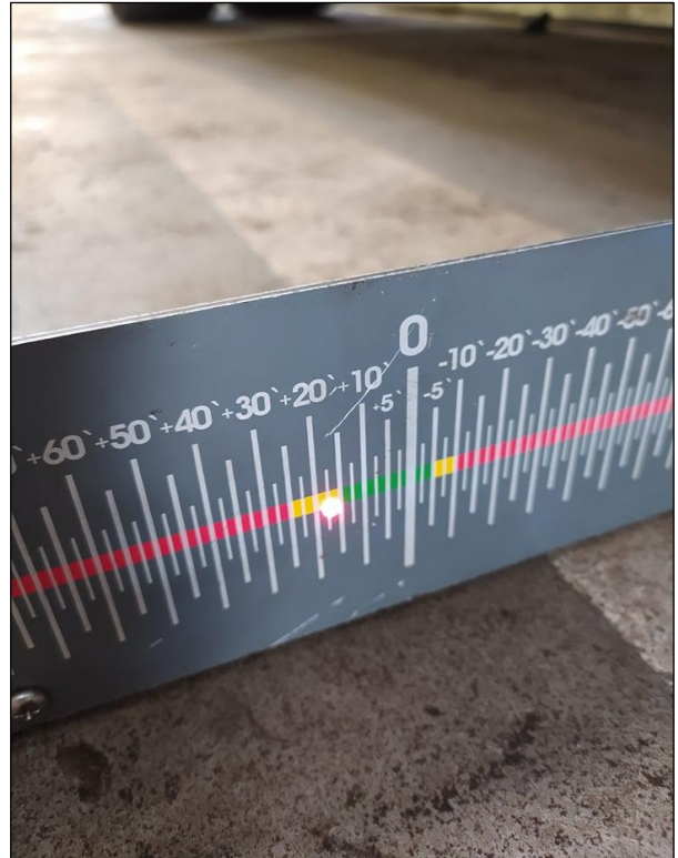
Obr. č. 47: Odchylnka předních kol [vlastní]
