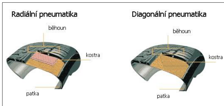
Obr. č. 10: Radiální a diagonální pneumatika [6]
