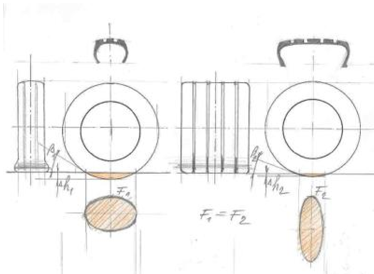
Obr.6.8 Porovnání širokého a úzkého pláště
