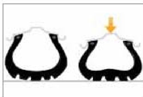
Obr.1.2.4 Radiální pláště
