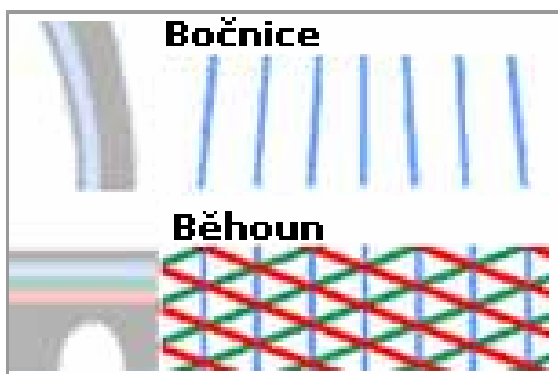
Obr.3.3 Vlákná radiálního pláště
