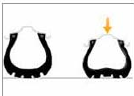
Obr.1.2.3 Diagonální pláště
