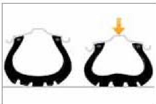
Obr.3.5 Zatížený a nezatížený radiální plášť
