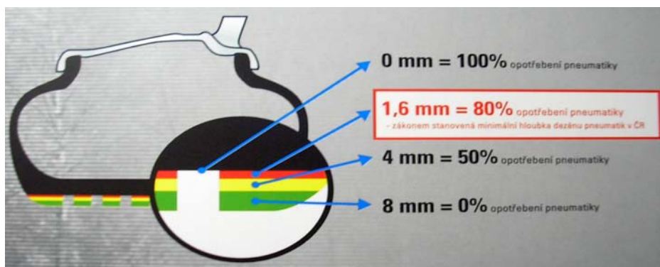
Obr. 6.6 Opotřebování dezénu
