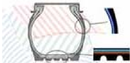
Obr.3.2 Vyztužení bočnic
