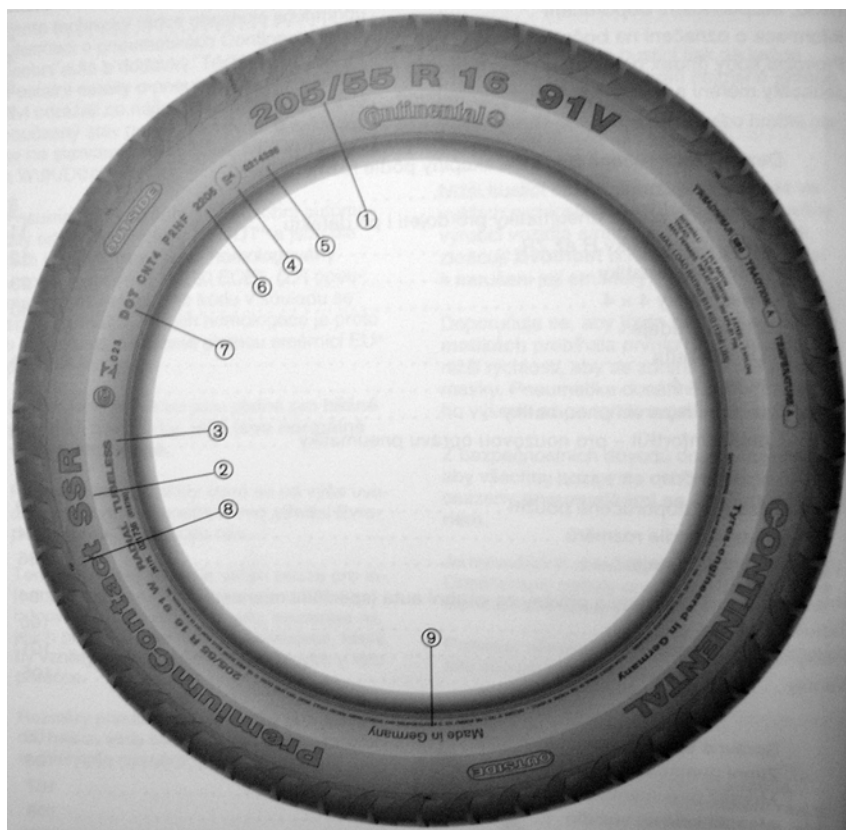
Obr.2.1 Popis pláště
