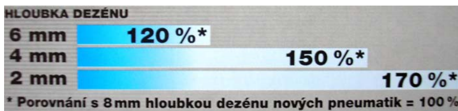
Obr. 6.7 Porovnání brzdné dráhy – zimní pláště na zasněžené vozovce
