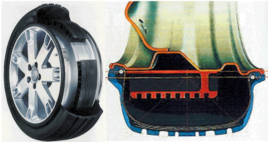
Obr. 8.1 Systém PAX
