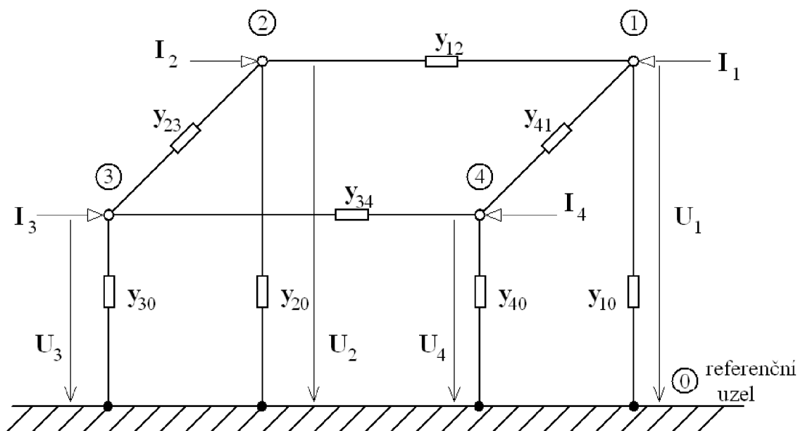
Obr. 2-1 Náhrada prvků sítě podélnými a příčnými admitancemi
