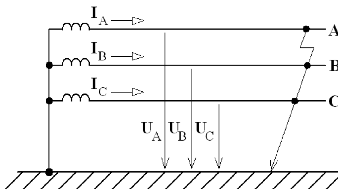
Obr. 2-11 Trojfázový zemní zkrat
