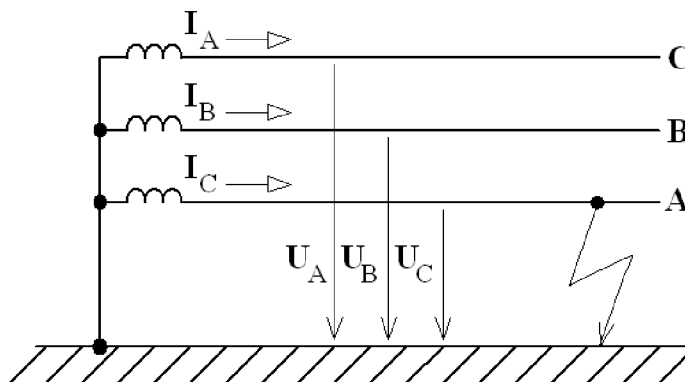
Obr. 2-12 Jednofázový zkrat
