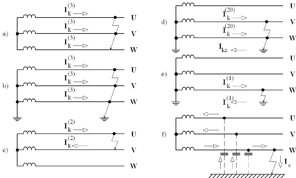
Obr. 2-7 Druhy zkratu
