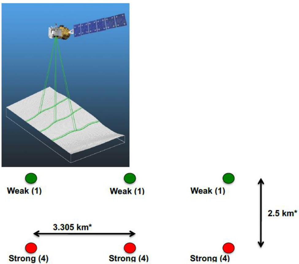
Obrázok 3: Schéma laserovej konfigurácie pre misiu ICESat-2. Energia je rozdelená do 3 párov laserových lúčov- vždy je jeden slabý a jeden silný. (Prevzaté z Neuenschwander et Pitts, 2021)
