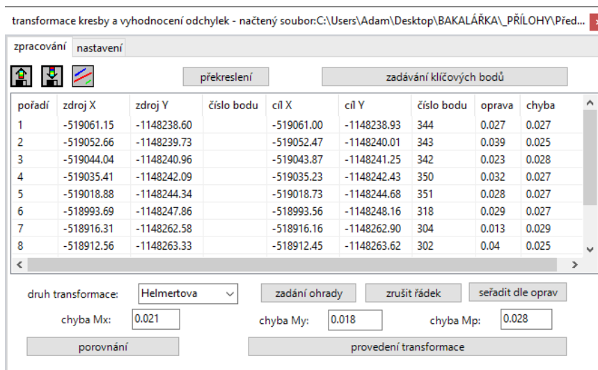
Obr. 15 Okno transformace kresby a vyhodnocení odchylek
