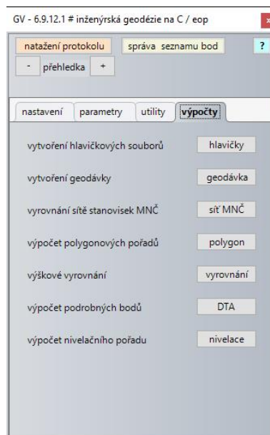
Obr. 12 GeoVýpočty – výpočty
