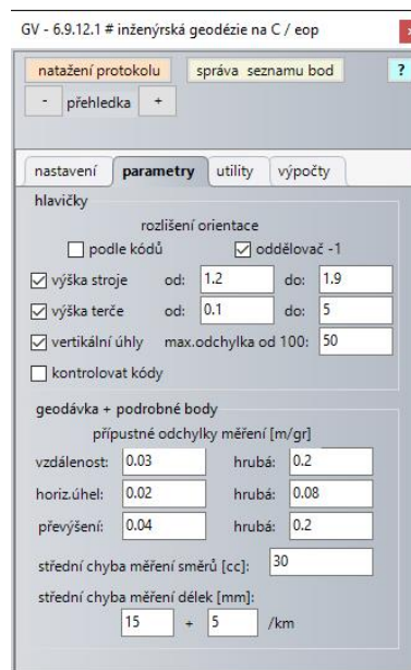
Obr. 8 GeoVýpočty – parametry
