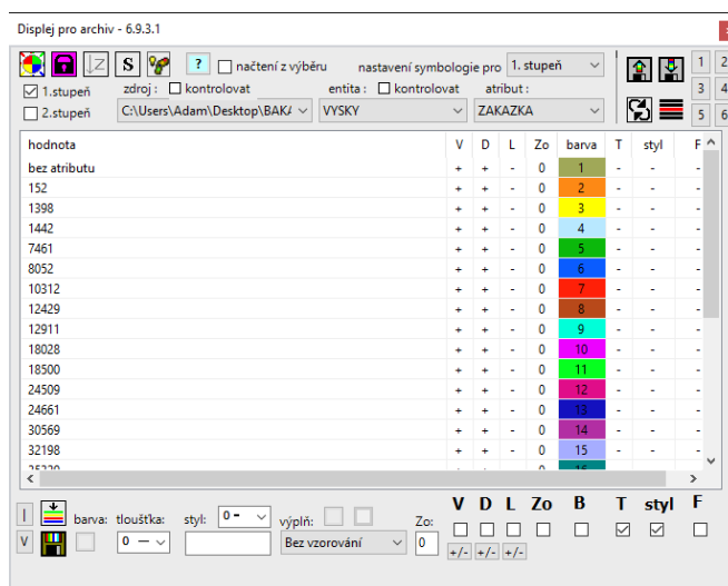
Obr. 14 Aplikace ADisplay
