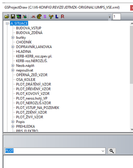
Obr. 25 Aplikace GSProjectDraw
