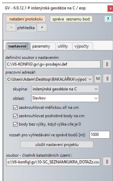
Obr. 7 GeoVýpočty – nastavení
