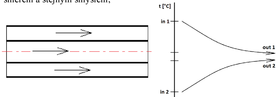
Obrázek 1.4 Souproudý výměník
