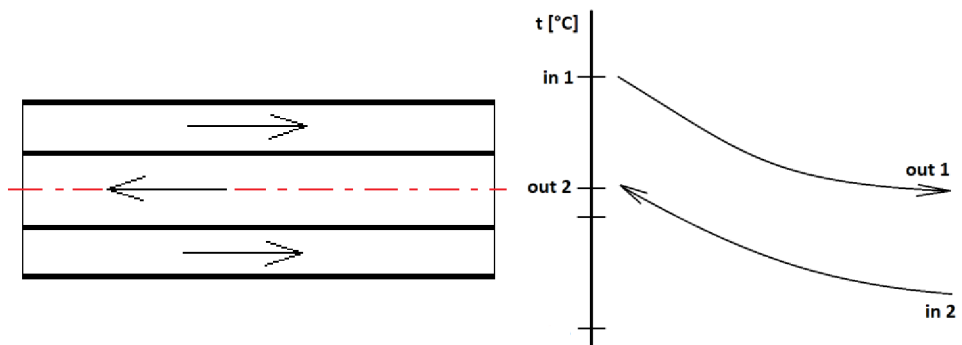
Obrázek 1.5 Protiproudý výměník
