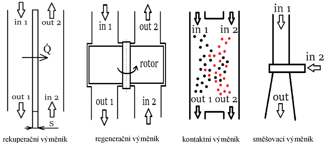
Obrázek 1.2 Typy výměníků
