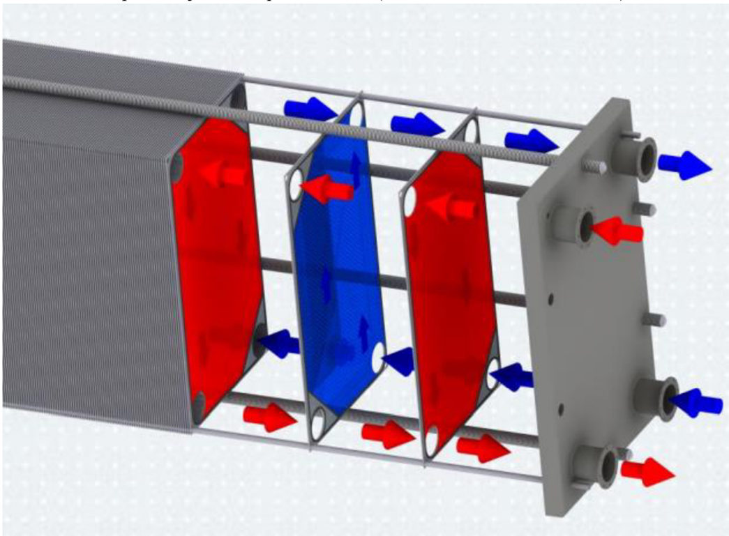
Obrázek 1.13 Proudění v deskovém výměníku [13]
