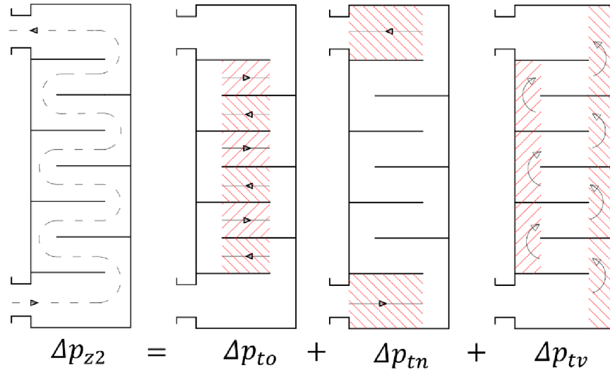
Obrázek 2.3. Schéma tlakových ztrát v jednotlivých úsecích MP
