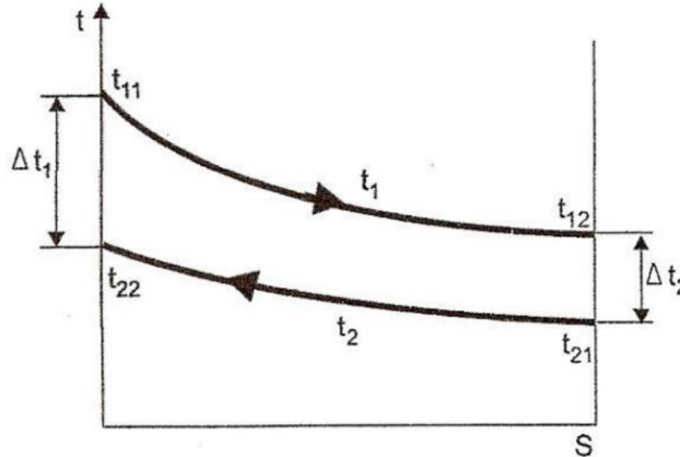
Obrázek 2.2 Změna teplot při výměně tepla, protiproud
