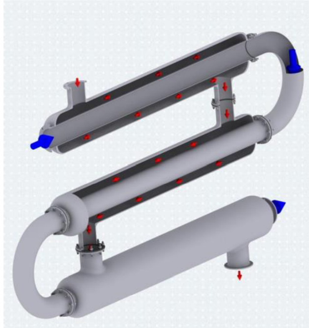
Obrázek 1.9 Článkový, dvoutrubkový výměník tepla [13]
