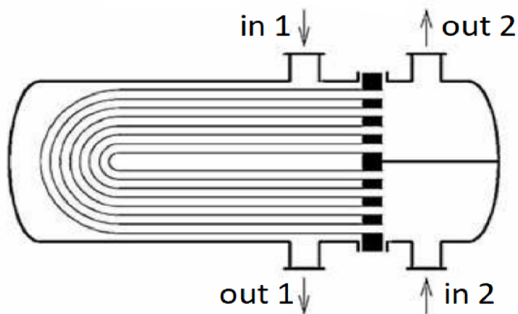
Obrázek 1.10 Schéma výměníku s U-trubicemi [10]
