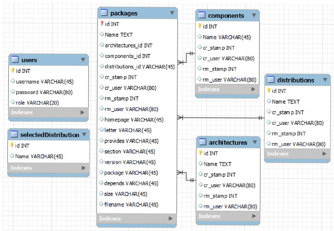
Obrázok 6 : Štruktúra databáze
