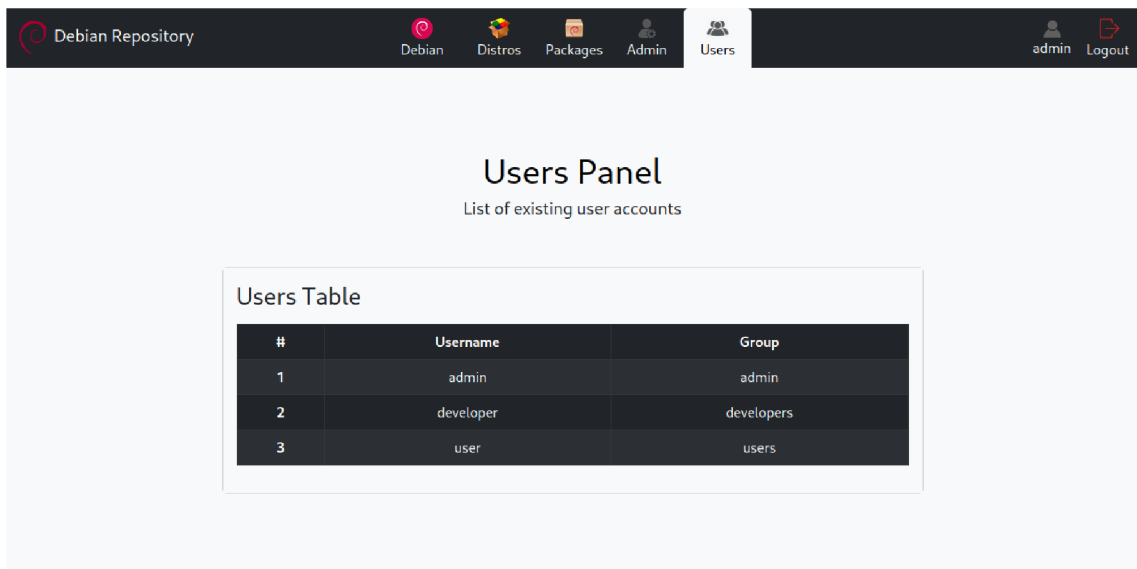
Obrázok 13 : Users Panel
