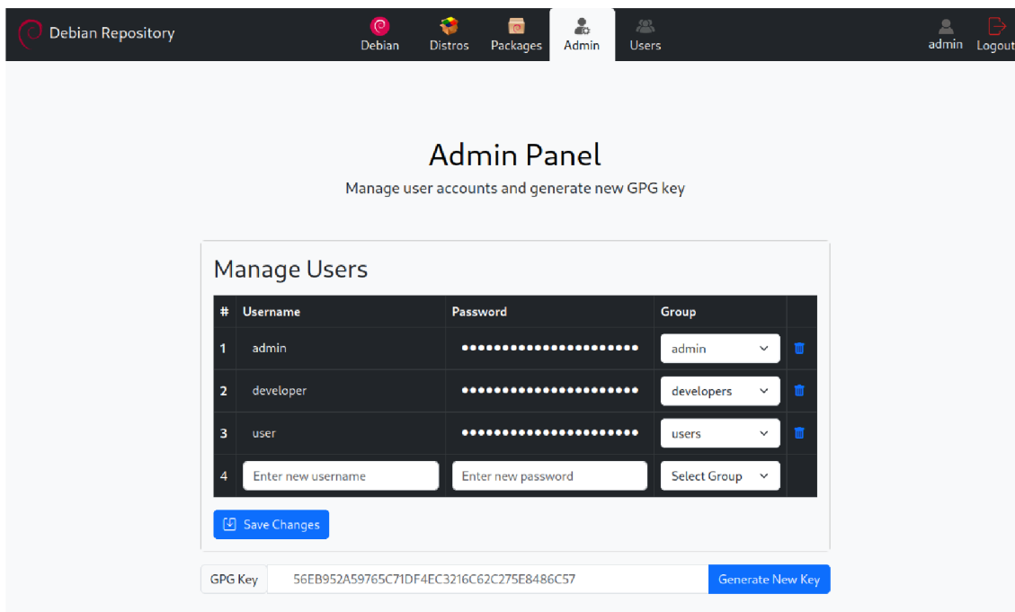
Obrázok 11 : Admin Panel
