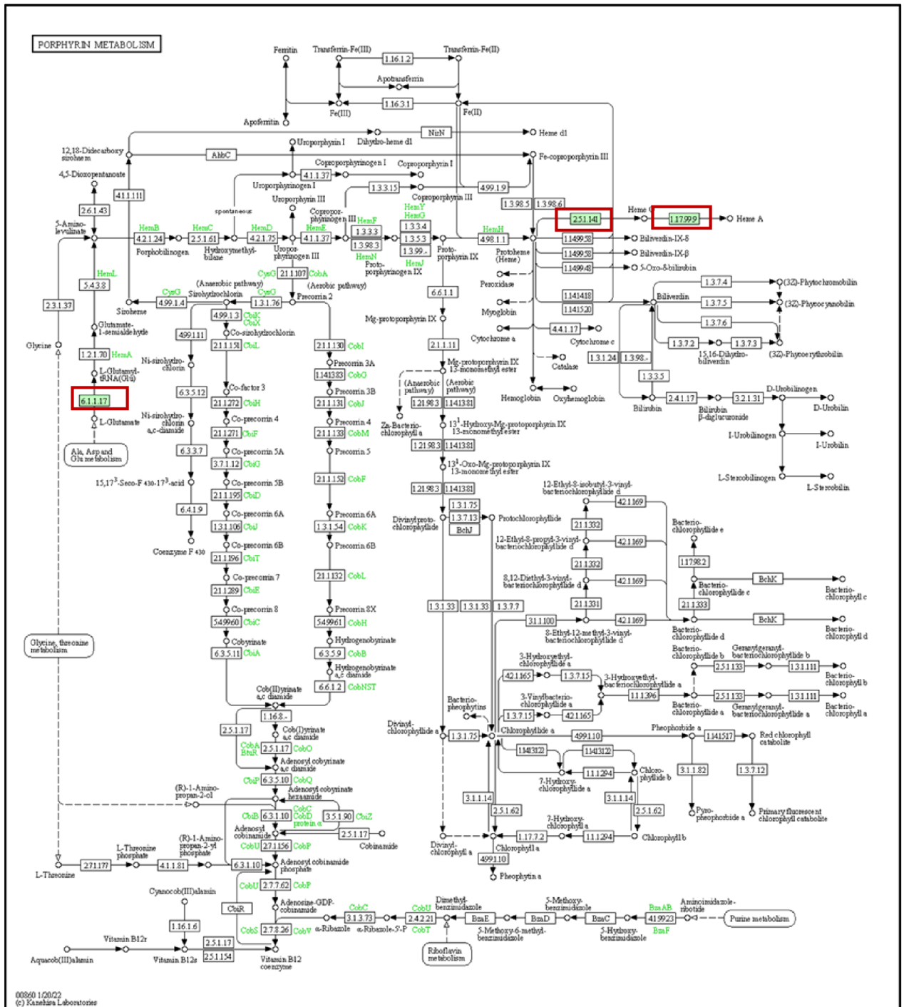
Obr. 3: Enzymy Glutamyl-tRNA synthetase, Heme A synthase a Heme O synthase (červeně zvýrazněné) v metabolismu porfyrinu u bakterie L. polyplacis .
