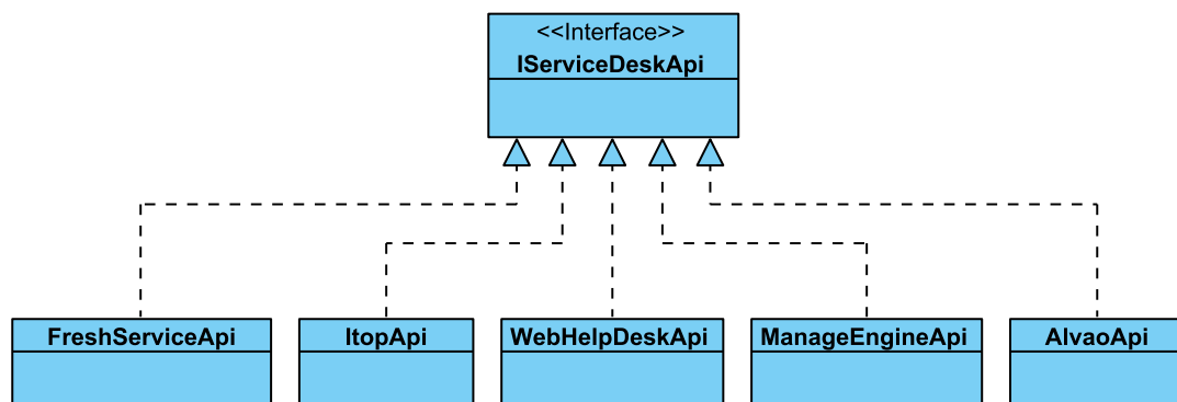
Obrázek 5.2: Model rozhraní. Zobrazuje konkrétní vnitřní klienty rozhraní (klienti webových služeb konkrétních SD systémů).
