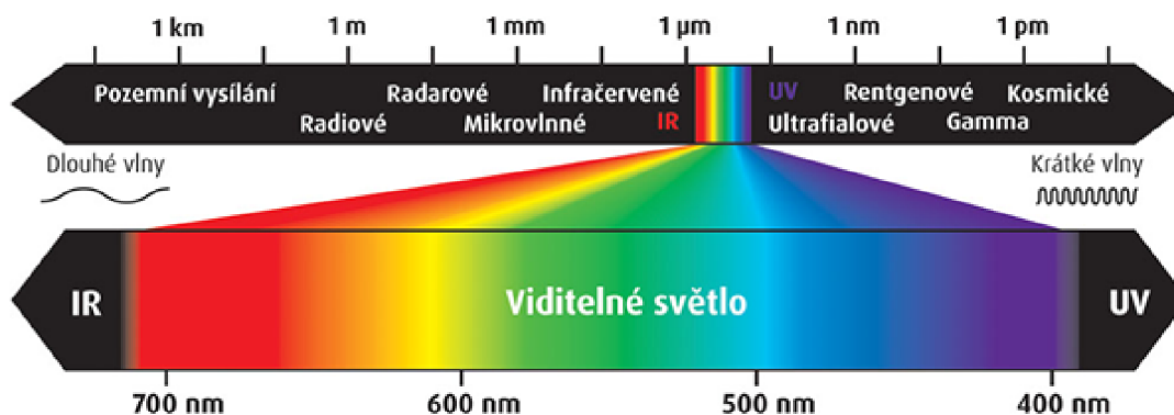
Obr. 1.1: Spektrum záření [2].
