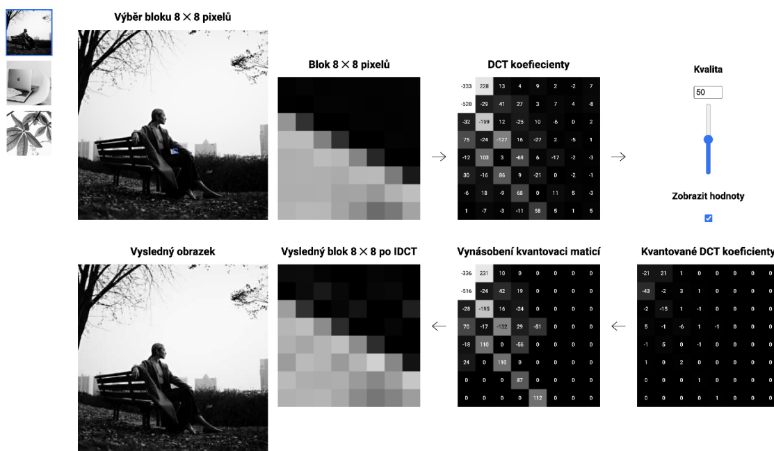
Obr. 2.5: Ukázka appletu „Ilustrace efektu změny DCT koeficientů na vzhled obrazu“.
