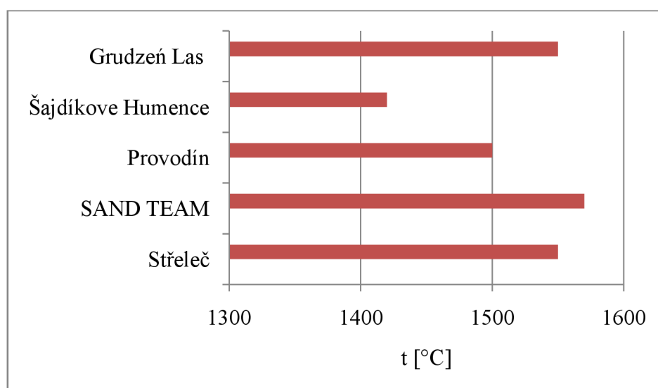
Graf 1 Počátek spékání jednotlivých křemenných ostriv.
