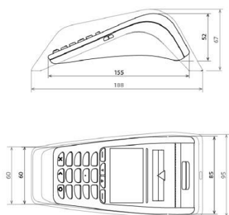
Základní rozměry rámu a terminálu M (1:1)
