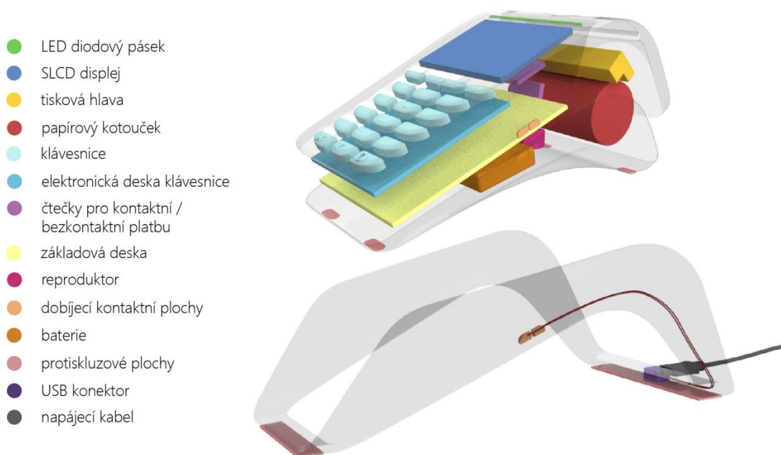
Obr. 6-1 Uspořádání vnitřních komponent přístroje
