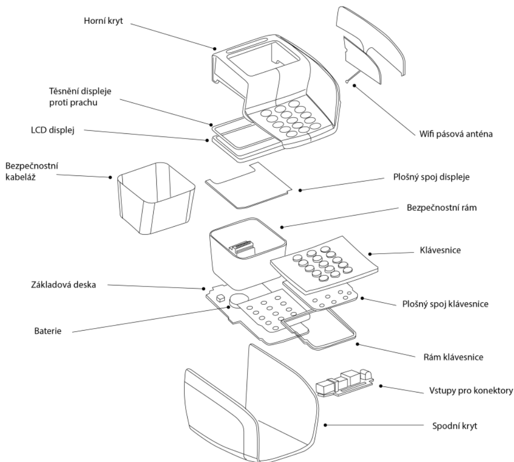
Obr. 2-12 Zobrazení technických částí terminálu Yomani BU (upraveno) [25]
