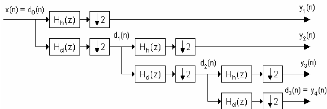
Obr. 1.5 Přímá rychlá DTWT pro tři úrovně rozkladu.
