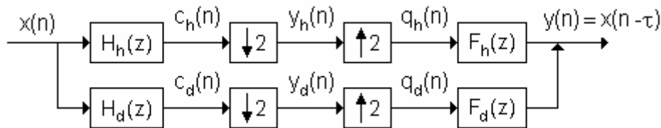
Obr. 1.7 Dvoukanálová banka rozkladových ( H_d, H_h ) a rekonstrukčních ( F_d, F_h ) filtrů.
