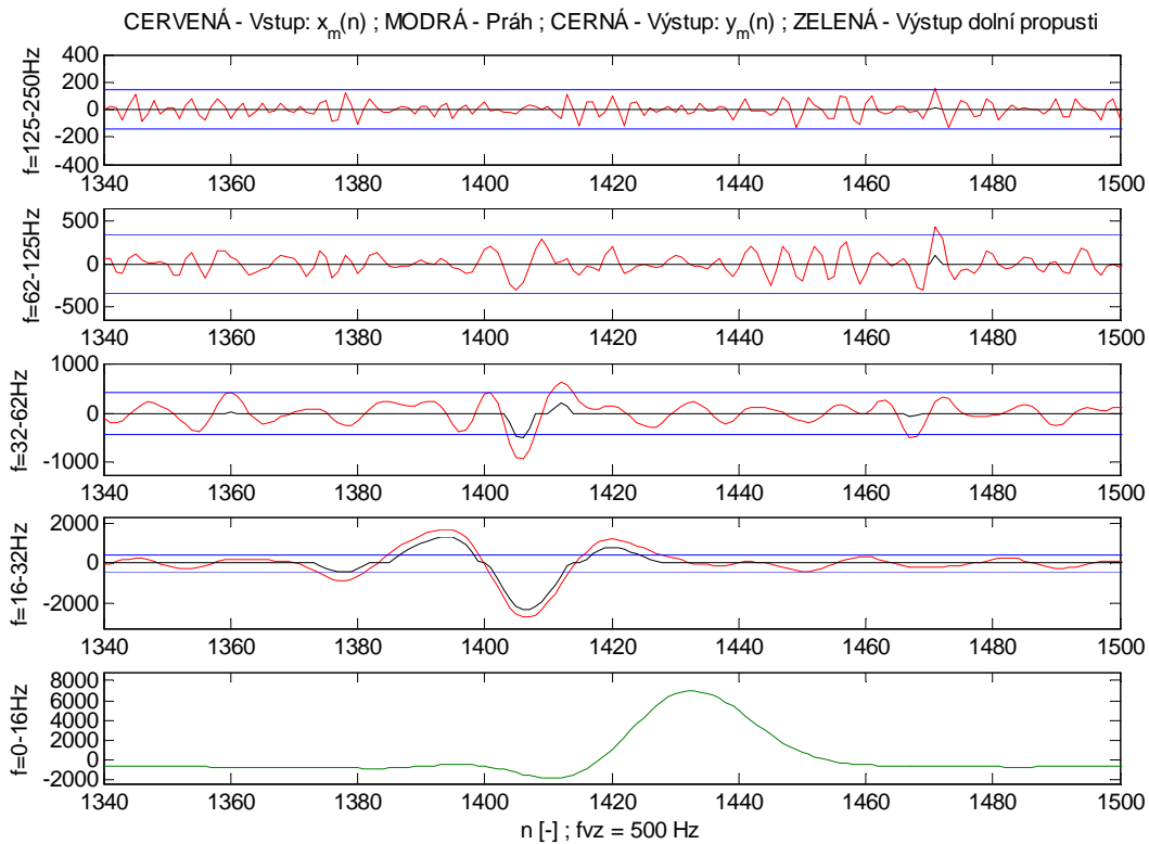
a) Červená - Vstupní rušený signál rozložený do frekvenčních pásem; Modrá - Prahy v jednotlivých pásmech; Černá - Signál po prahování; Zelená - Výstup dolní propusti.
