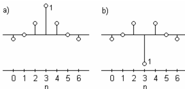
Obr. 1.8 Příklad impulsní charakteristiky zrcadlových filtrů P_d(z) a P_h(z) .
