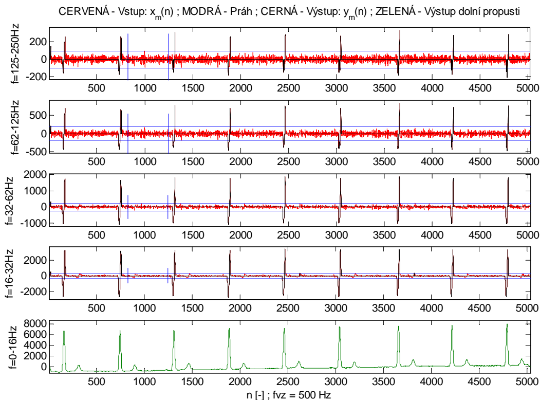
Obr. 3.3 4-stupňový rozklad EKG signálu + Výstup dolní propusti.
