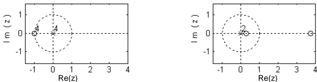
Obr. 1.11 Rozložení nulových bodů pro 4 varianty dvojic rozkladových a rekonstrukčních dolních propustí odvozených z půlpásmového filtru {}^3P_d(z) .
