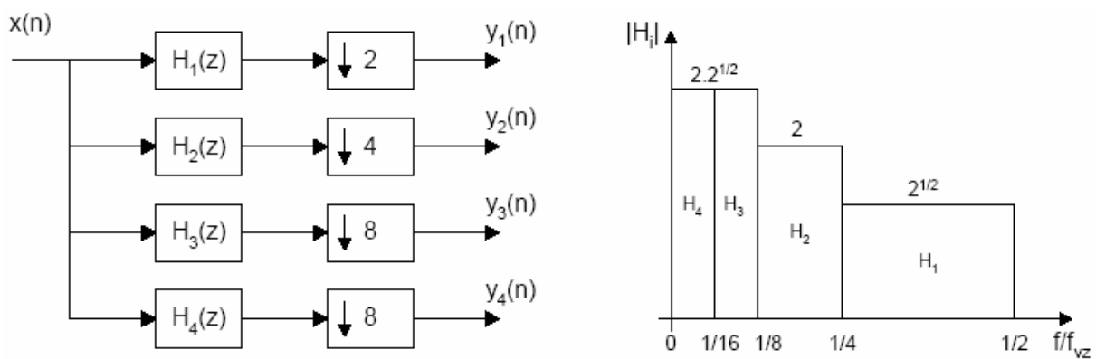
Obr. 1.3 Vlevo: realizace třístupňové dyadické DTWT bankou oktákových filtrů s podvzorkováním výstupů. Vpravo: modulové frekvenční charakteristiky ideálních oktákových filtrů.
