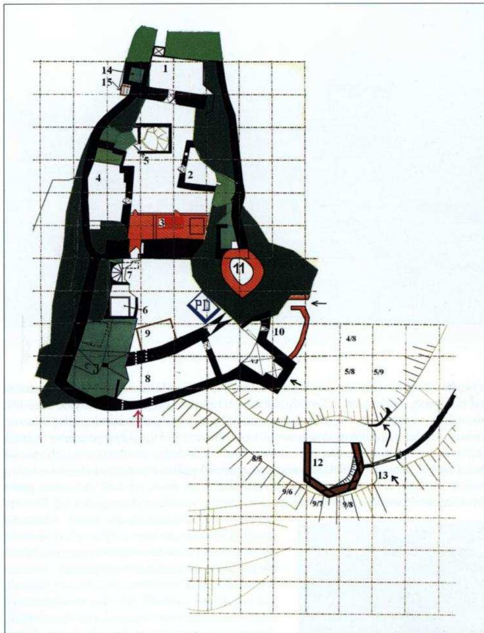
Obr. 2. Půdorys hradu Skály. Legenda: barvy: černá – zdivo, zelená – skály, světle zelená – skály začleněné do obytných a provozních prostor, oranžová – dodatečné stavby po roce 1425, 1 – palác, 2 – vstup na věž a hrady, 3 – nová kuchyně, 4 – tzv. purkrabství, 5 – cisterna, 6 – původní kuchyně, 7 – schodiště, 8 – stáje, 9 – kolna na postroje, 10 – bastion, 11 – břítová věž, 12 – obranný srub na valu, 13 – černé šipky – směr ustupu, vstupní brána, 14 – severovýchodní věž, 15 – prevet, VJ – vlcí jáma, PD – penězokazecská dílna, J – jeskyně, fialová šipka – směr útoku, prolomení hradeb (zaměření D. Šiler).
