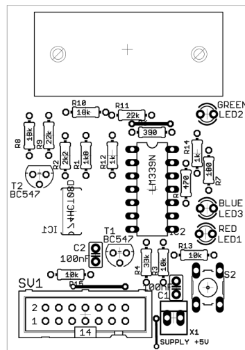
Príloha 6: Osadzovací plán plošného spoja pre rozširujúcu dosku bluetooth modulu
