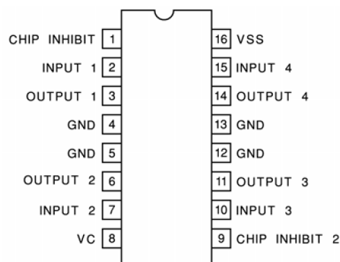
Obr. 3.12: Rozloženie nožičiek obvodu L293B
