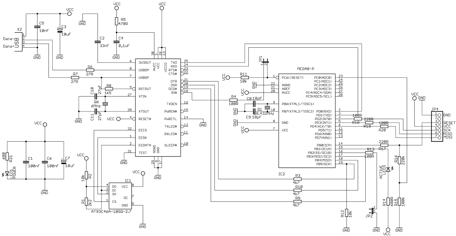
Príloha 8: Schéma zapojenia USB programátora pre AVR
