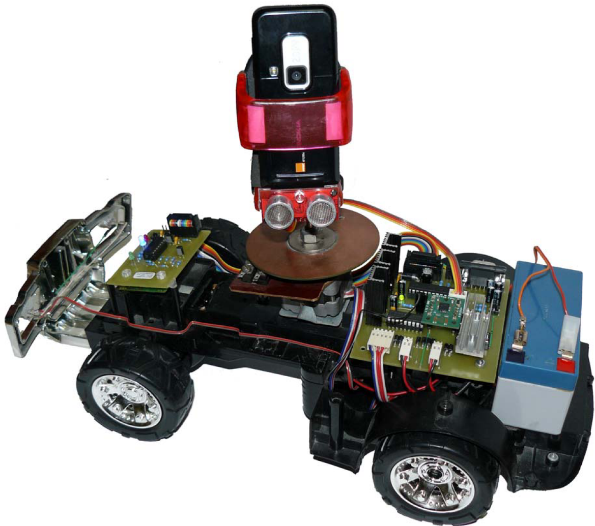
Príloha 14: Celkový pohľad na mobilmú platformu
