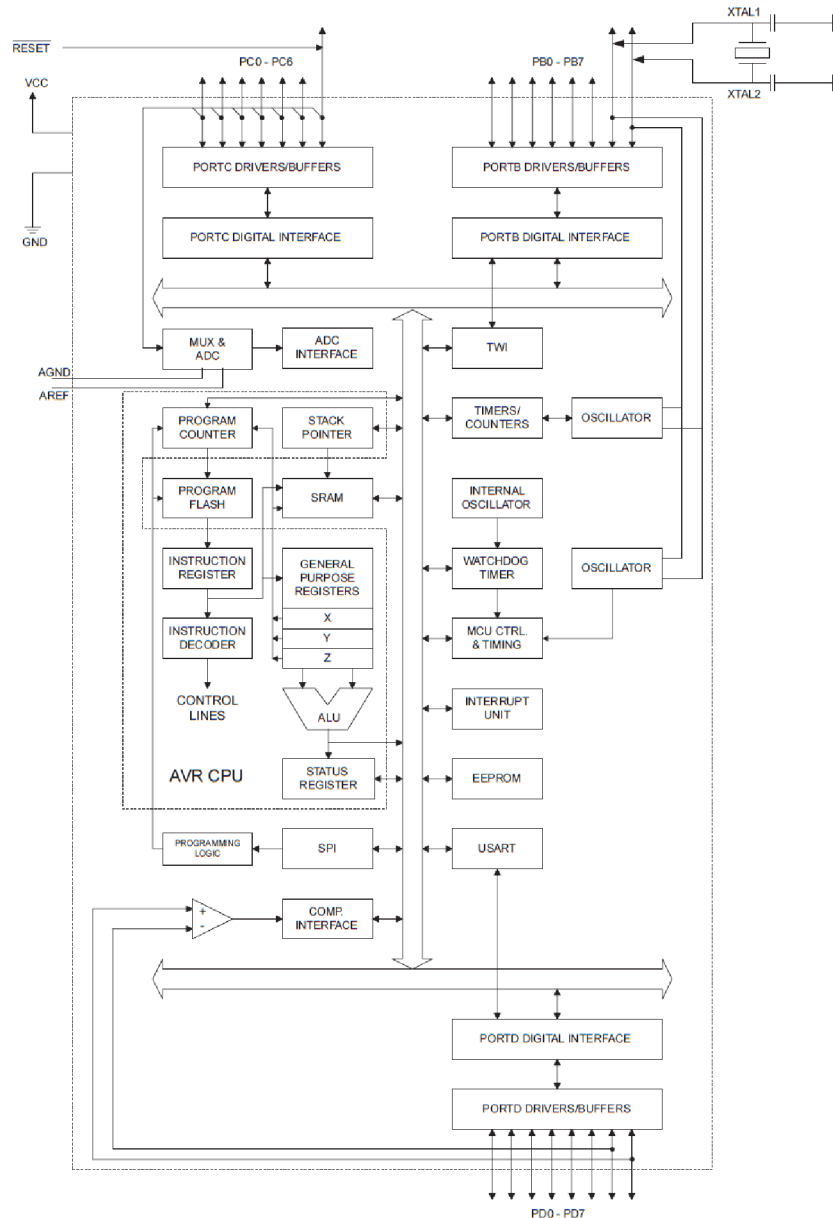
Obr.2.1: Bloková schéma ATmega 8
