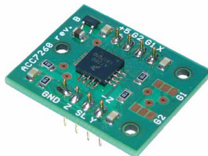
Obr. 3.14: Trojosý akcelerometer ACC7260
