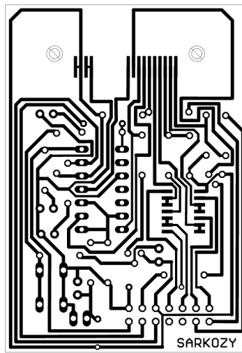
Príloha 5: Plošný spoj rozširujúcej dosky pre bluetooth modul
