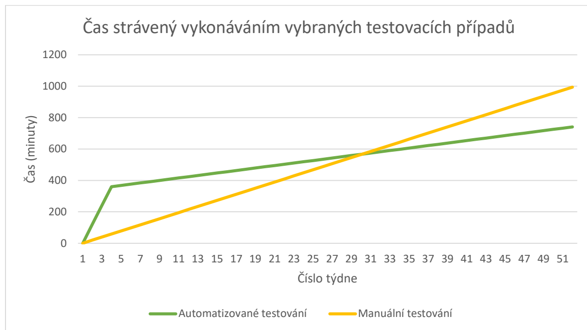
Tabulka 6 - graf ročního vývoje času stráveného nad manuálním a automatizovaným testováním
