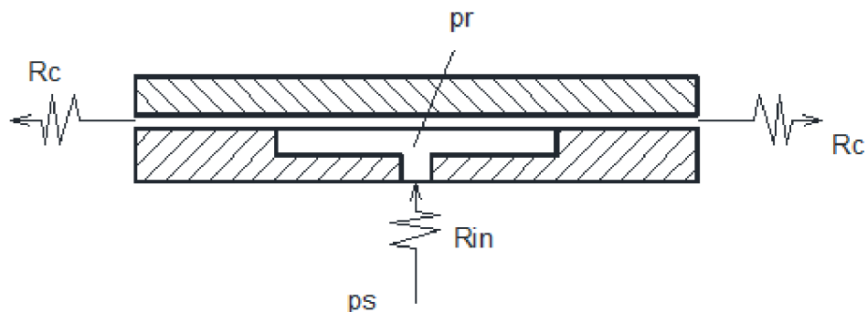
Obr. 21 - Hydrostatická buňka s vyznačenými odpory proti proudění
