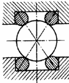
Obr. 12 - Drátové ložisko (6)
