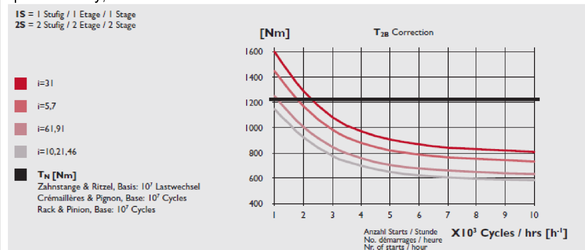
Obr. 28 - Závislost maximálního výstupního kroutícího momentu převodovky Gudel na počtu cyklů zrychlování a zpomalování
