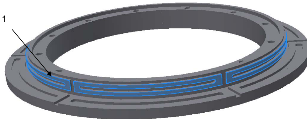
Obr. 42 - Model radiálního hydrostatického ložiska
