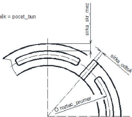
Obr. 39 - Skutečná a zjednodušená hydrostatická buňka axiální ložiska
