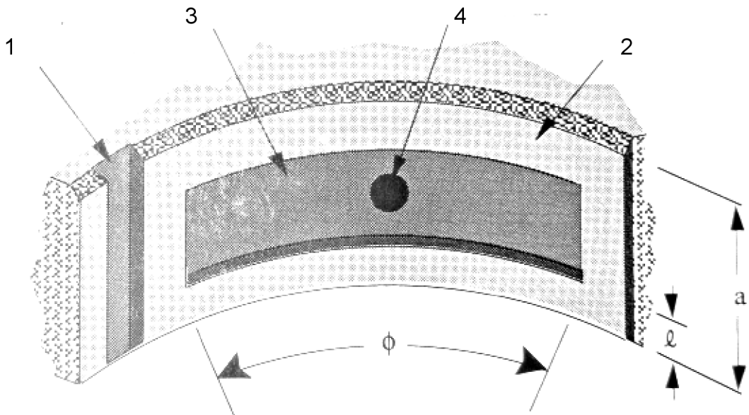
Obr. 24 - Hydrostatická buňka radiálního ložiska
