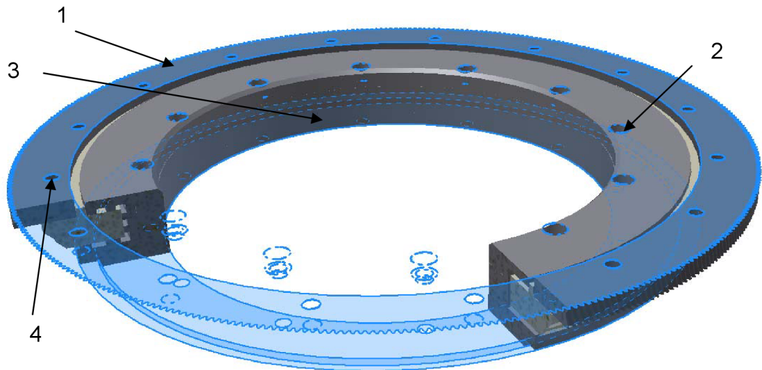
Obr. 33 - Pohled na model axiálně-radiálního ložiska a pohon otočného stolu
