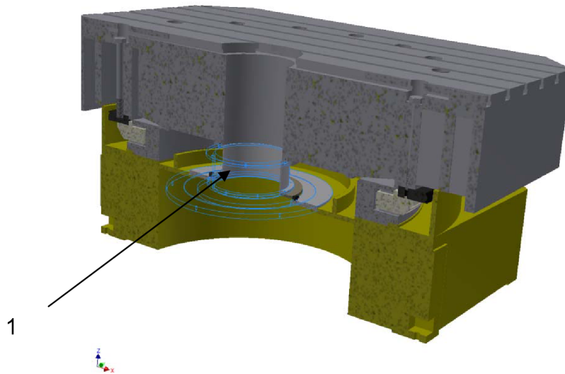
Obr. 51 - Odměřovací systém otočného stolu
