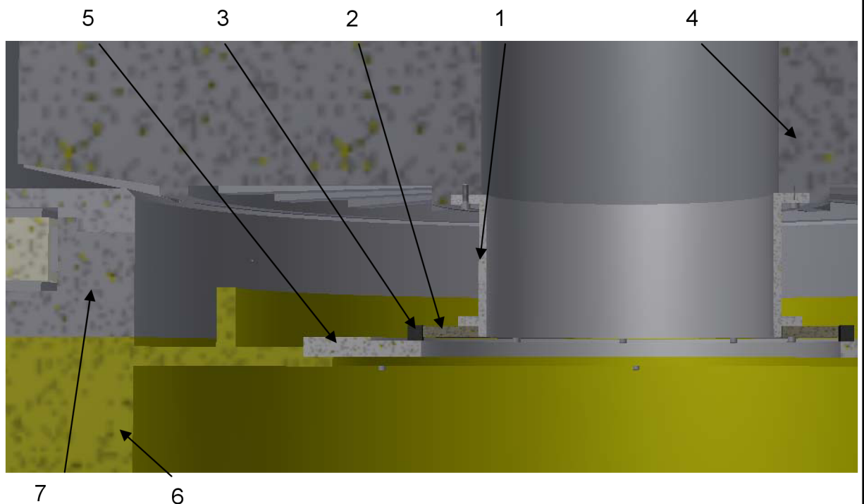
Obr. 52 - Uložení odměřovacího systému
