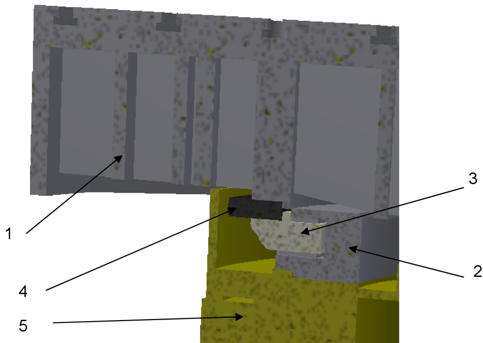
Obr. 47 - Detail uložení upínací desky
