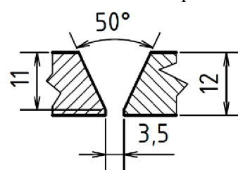
Obr. 23 Geometrie svarových ploch dle podnikové WPS
