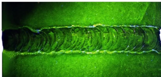
Obr. 27 Lícové strany vzorků při MT
