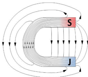
Obr. 8 Orientace siločar MP u magnetu [23]
