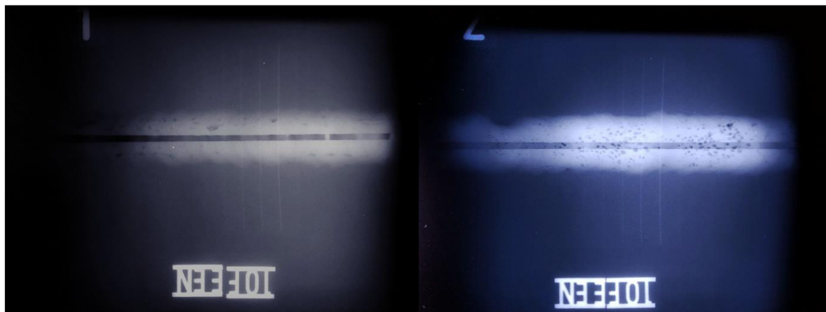
Obr. 29 Radiogramy svarů
