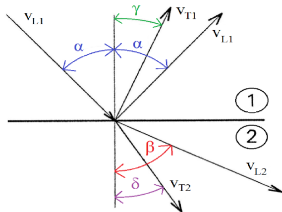
Obr. 13 Rozhraní prostředí [1]
