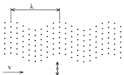
Obr. 12 Příčné vlnění [1]
