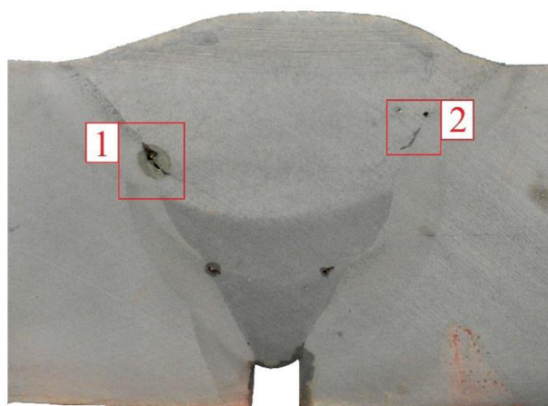
Obr. 34 Vybroušené a naleptané vzorky
