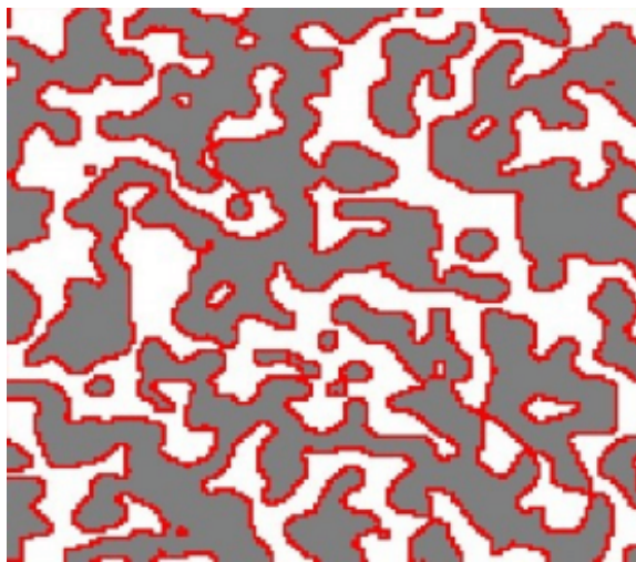
Obrázek 2.7: Jeskyně složená z 9 mřížek o velikosti 50x50 buněk a vygenerovaná pomocí celulárního automatu. Šedě znázorněné jsou skály, bíle podlahy a červeně stěny. Použité parametry: r = 50\% , n = 4 , T = 13 , M = 2 . Převzato z [11].
