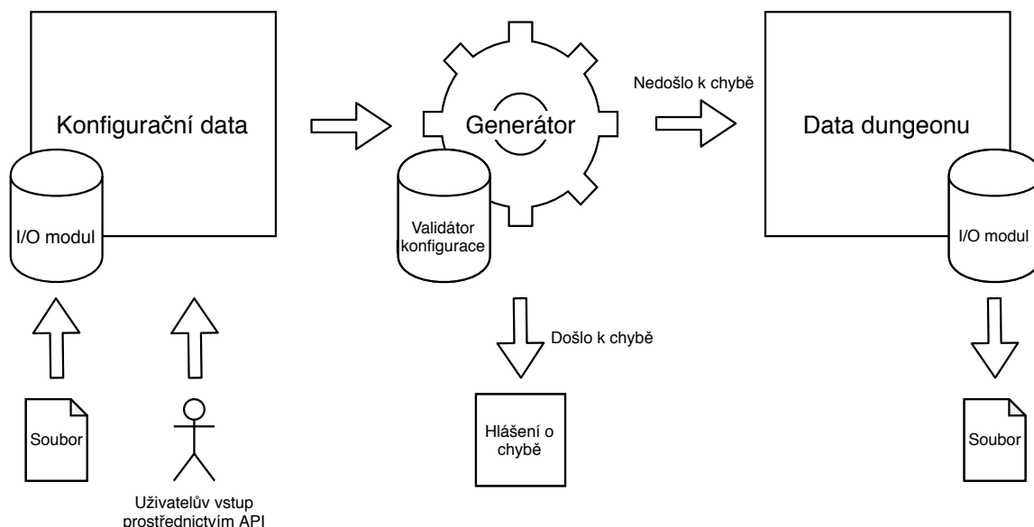
Obrázek 4.1: Obecný návrh struktury knihovny – knihovna načte konfigurační data (ať už zadaná uživatelem prostřednictvím API nebo jako soubor), tato data poté předá generátoru, který konfiguraci prověří a vygeneruje dungeon, který lze poté také převést do souborové podoby.
