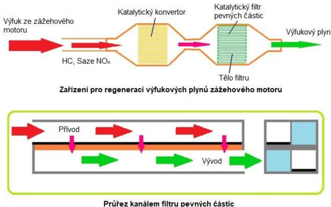
Obr. 12 Funkce a složení filtru pevných částic [37]
