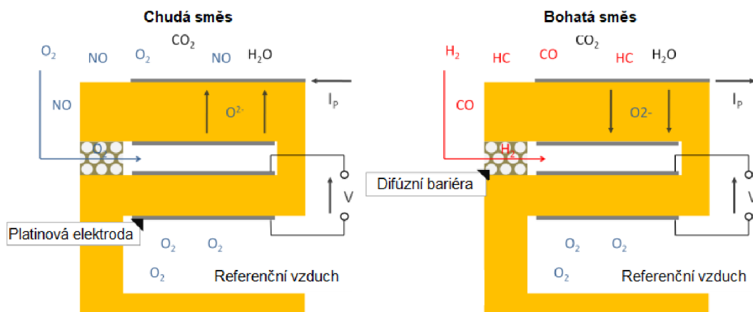
Obr. 8 Funkce lambda sondy na základě přenosu iontů kyslíku [31]
