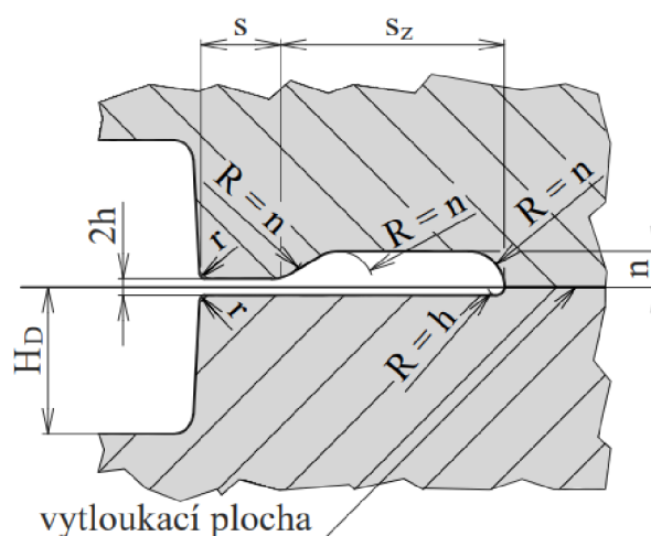
Obr. 27 Obvyklá výronková drážka pro buchar se zakotovanými rozměry
