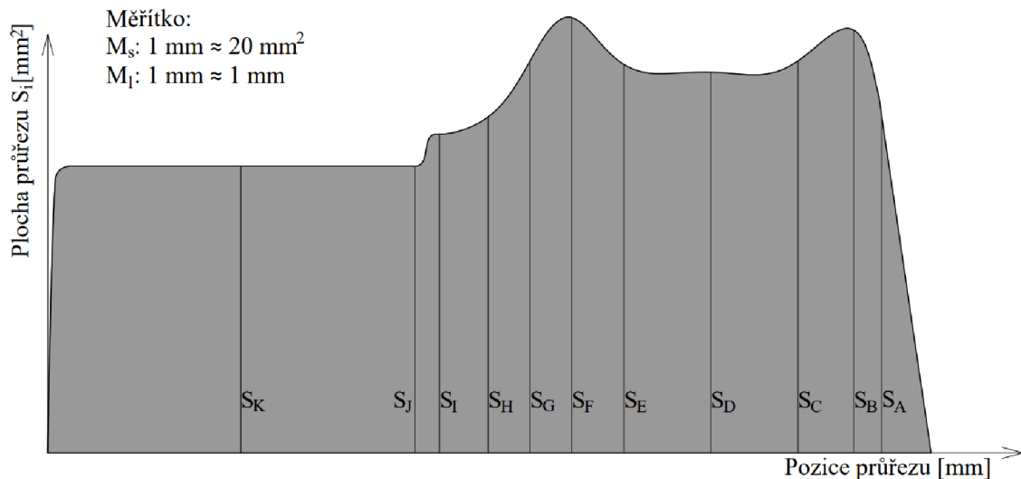
Obr. 29 Průřezový obrazec
