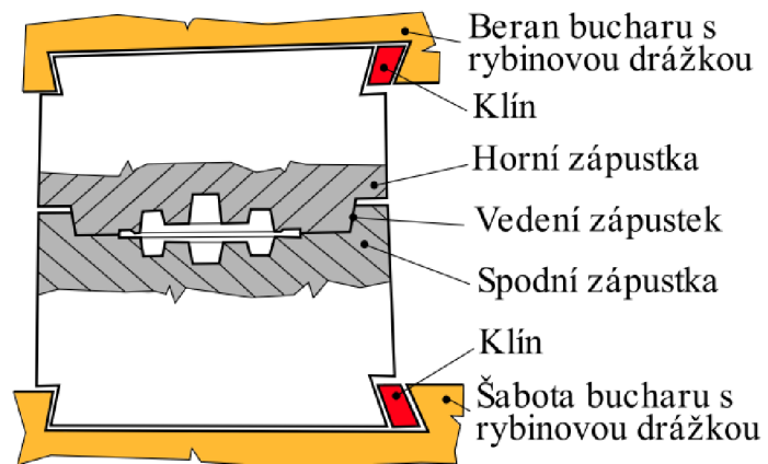
Obr. 20 Schéma upnuté zápustky bucharu [13]
