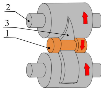
Obr. 23 Schéma PKV [20]
