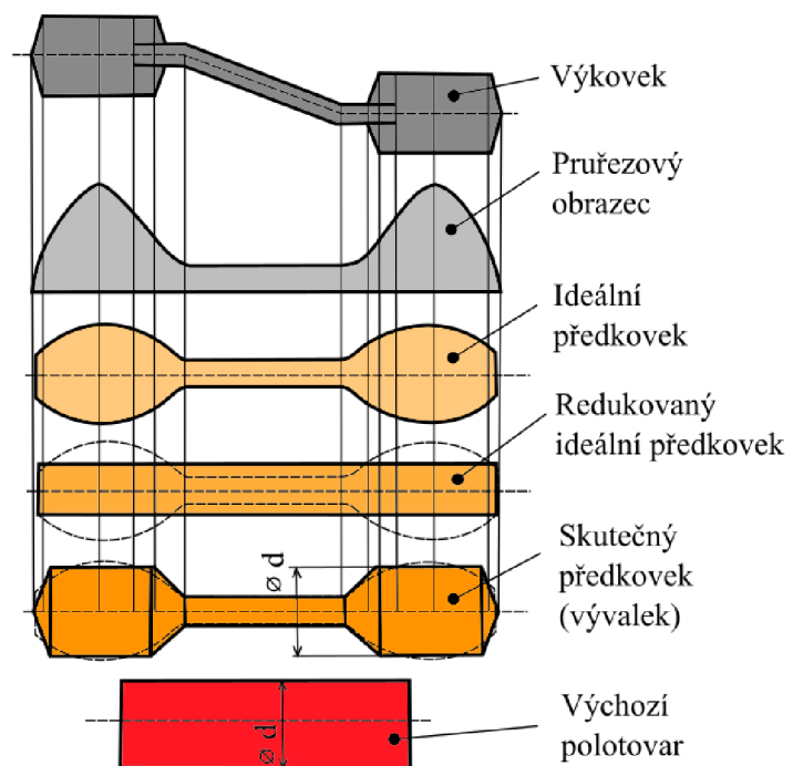
Obr. 22 Stanovení tvaru polotovaru složitějších výkovků [13]
