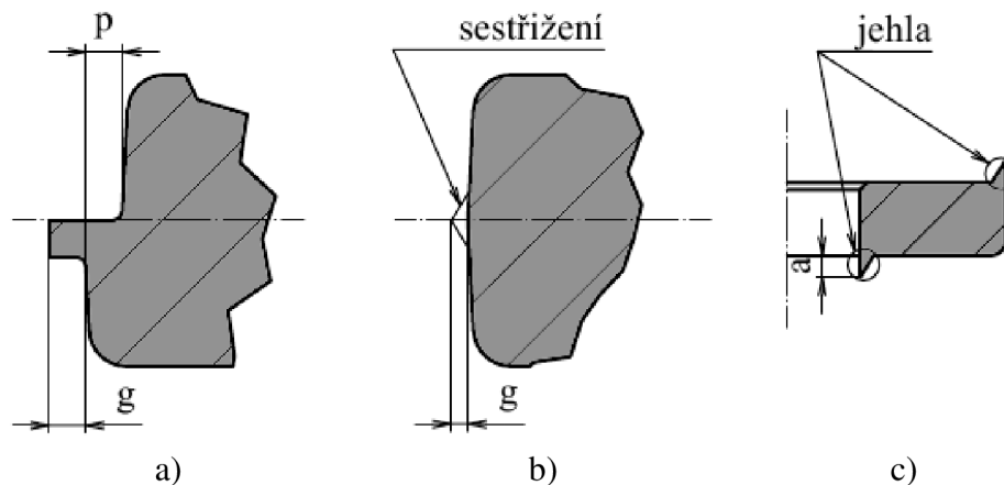
Obr. 16 Tvarové úchylky [26]
