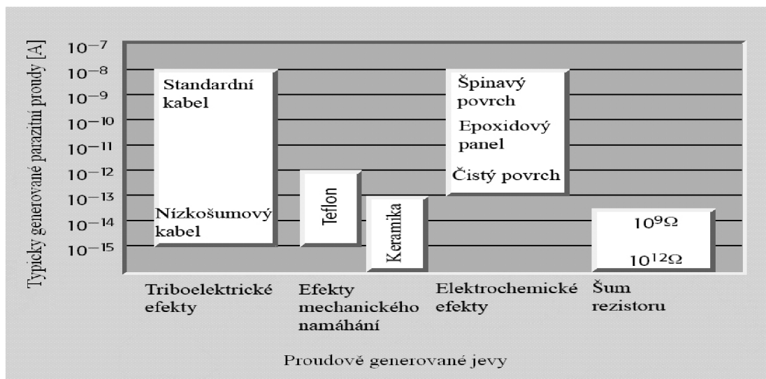
Obr. 6. : Velikosti proudů způsobujících chyby měření [11]
