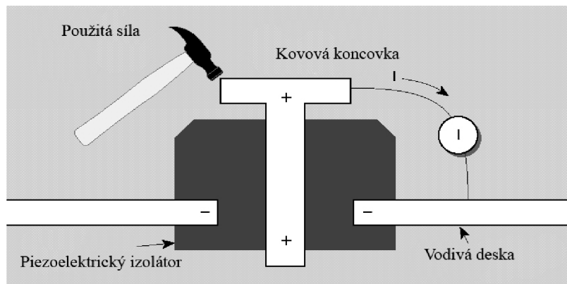
Obr. 8. : Piezoelektrický efekt [11]
