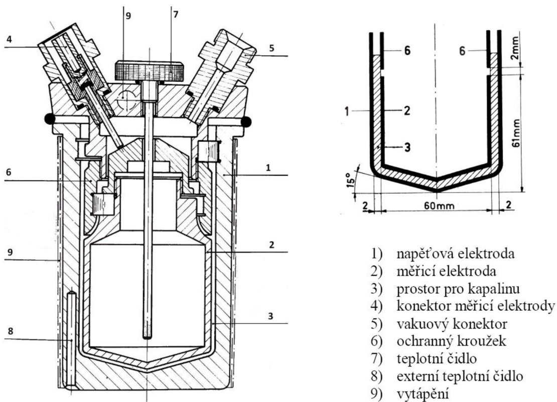
Obr. 11. Vnitřní schéma měřicího systému 2903 [16]
