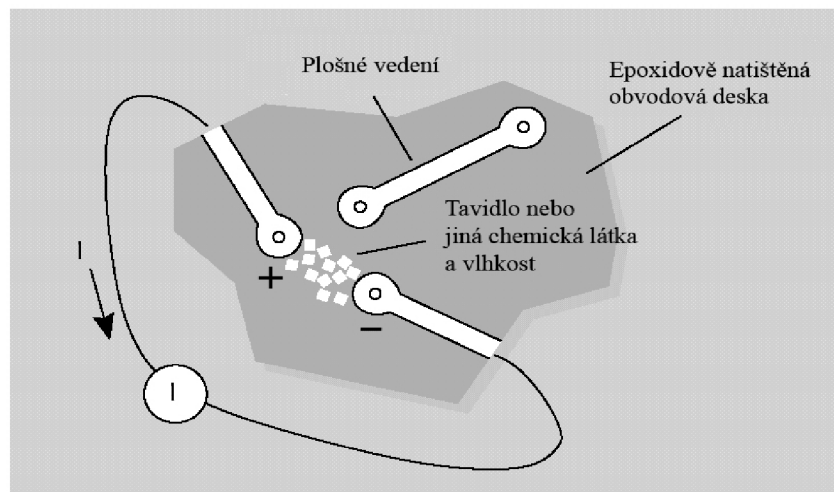
Obr. 9. : Chemický efekt [11]
