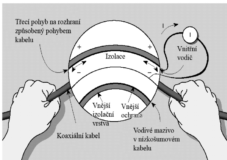
Obr. 7. : Triboelektrický efekt [11]
