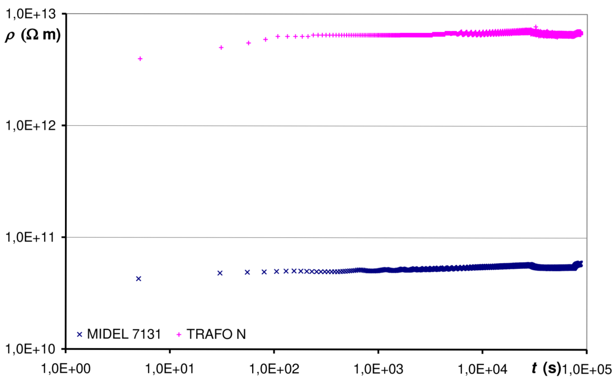
Obr. 26. Závislost vnitřní rezistivity na čase při teplotě 40^\circ \text{C}
