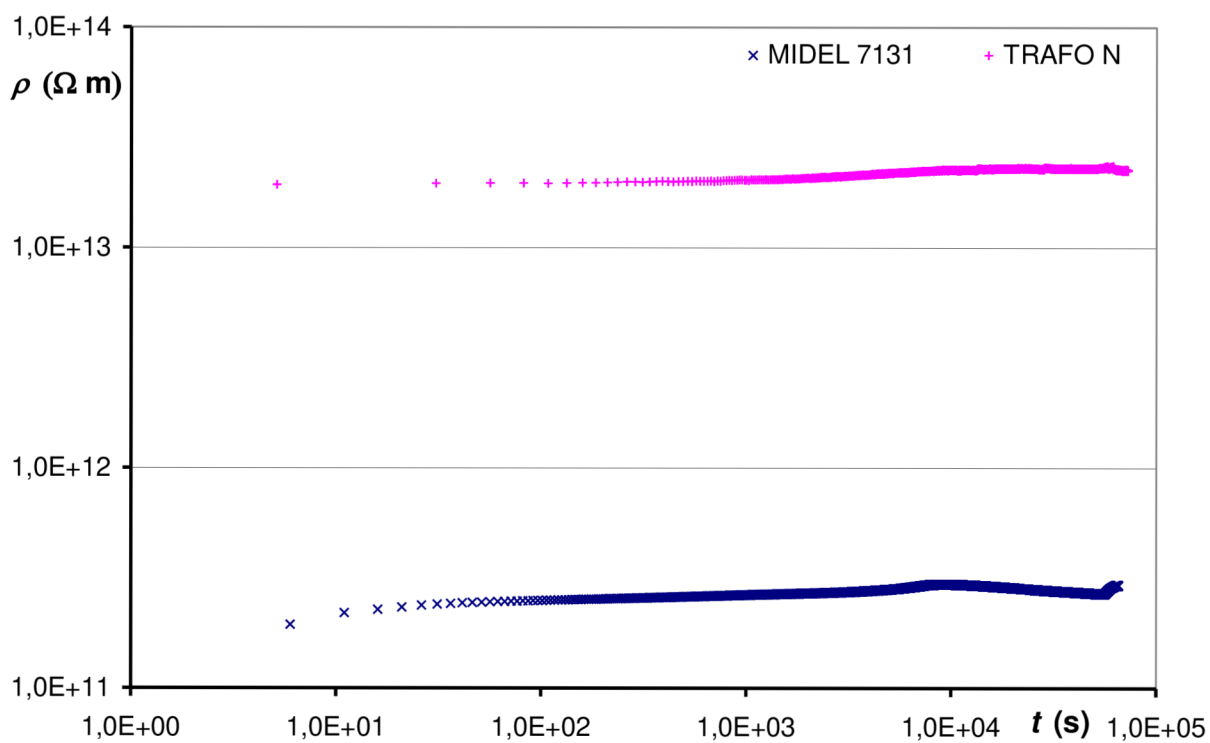
Obr. 25. Závislost vnitřní rezistivity na čase při teplotě 20^\circ \text{C}
