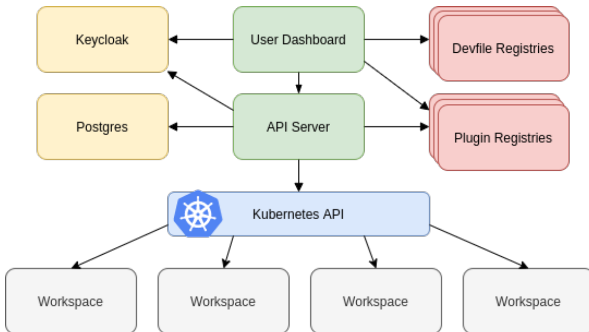
Obr. 2.2: Architektúra bloku Workspaces Controller. Ak je integrované programovacie prostredie Eclipse Che nasadené v móde jedného užívateľa, blok Keycloak nie je aktívny. Ilustrácia bola prevzatá zo zdroja číslo [36].
