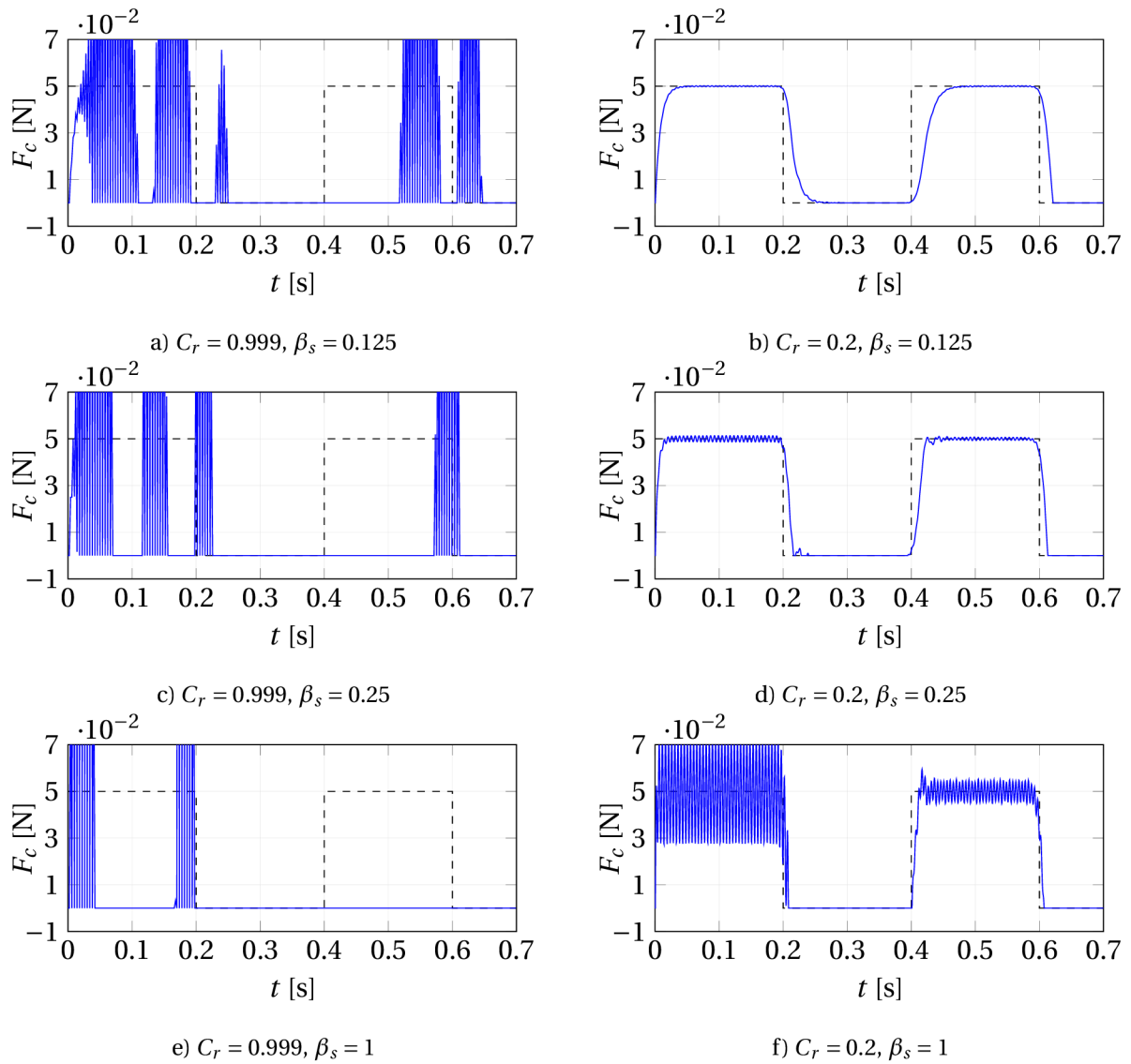
Obrázek 4.21: Výsledky kontaktní síly pro penaltovou metodu.
