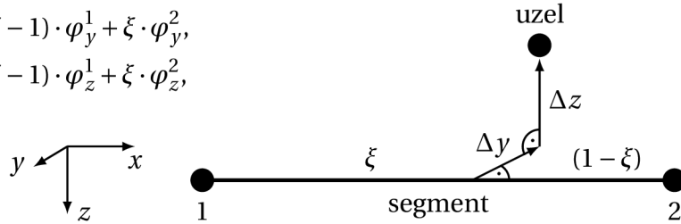
Obrázek 4.39: Geometrie relativního připojení uzlu na 1D segment.
