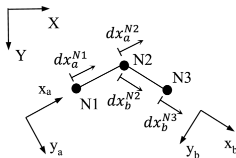
Obrázek 4.36: Element kladky [72].
