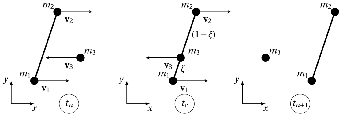
Obrázek 4.22: Penetrace kontaktu [74].
