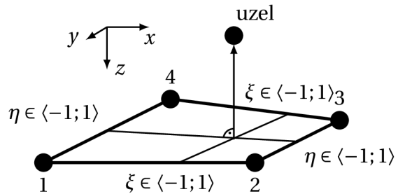
Obrázek 4.40: Geometrie relativního připojení uzlu na 2D segment.
