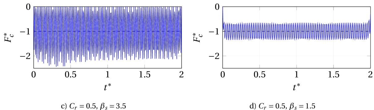
Obrázek 4.16: Výsledky kontaktní síly spočítané penaltovou metodou.
