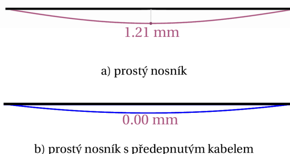
Obrázek 4.50: Výsledky průhybů.
