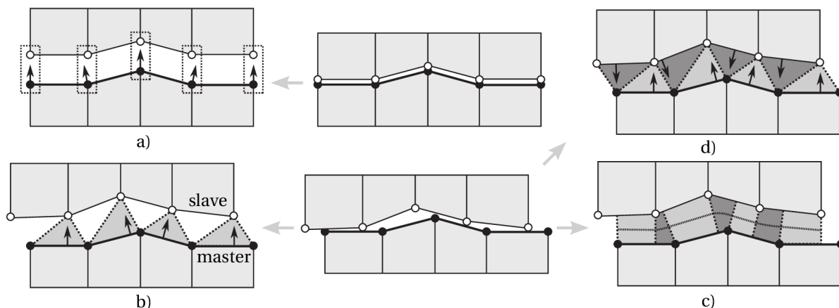
Obrázek 2.1: Znáornění různých druhů diskretizací kontaktů: a) node-to-node, dvojice uzlů a směr kontaktu; b) node-to-segment, slave uzly a jim příslušící master segmenty; c) segment-to-segment, kontaktní elementy a mezilehlá integrační linie; d) contact domain diskretizace, kontaktní elementy [63].
