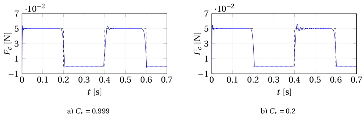
Obrázek 4.20: Výsledky kontaktní síly pro kinematickou metodu.
