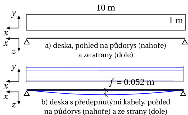
Obrázek 4.51: Znázornění dvou porovnávaných skořepinových modelů desky se statickým schématem prostého nosníku, kde varianta a) je pouze z betonu a model b) navíc obsahuje předpjaté kabely.
