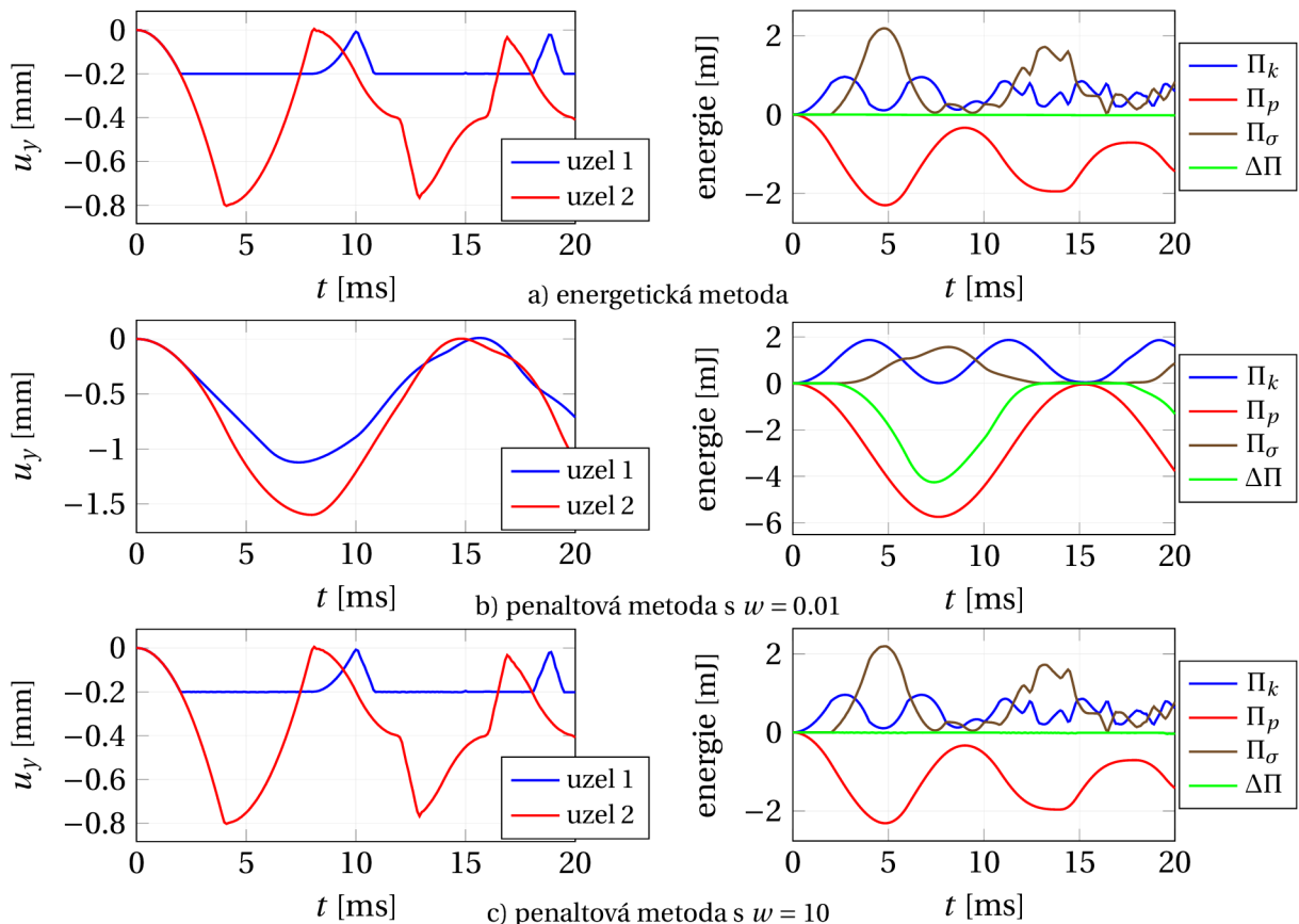
Obrázek 4.33: Deformace uzlů 1 a 2, společně s jednotlivými složkami energie pro energetickou metodu (a), penaltovou metodu s w = 0.01 (b) a penaltovou metodu s w = 10 (c).
