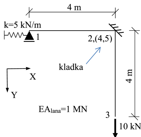
Obrázek 4.38: Příklad využívající element kladky [72].
