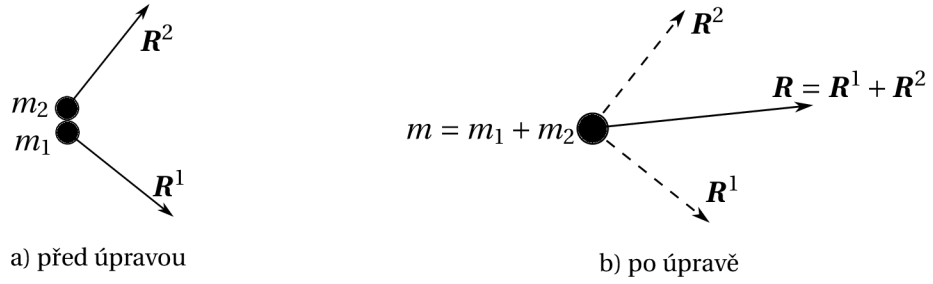
Obrázek 4.2: Ztotožnění sil a hmot.
