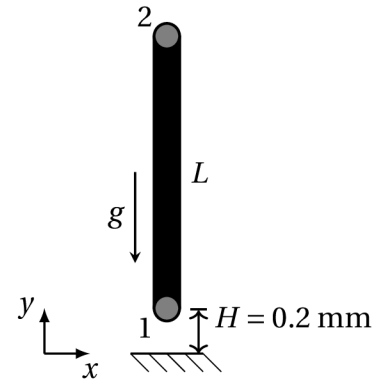
Obrázek 4.32: Elastický prut dopadající na tuhou podložku.
