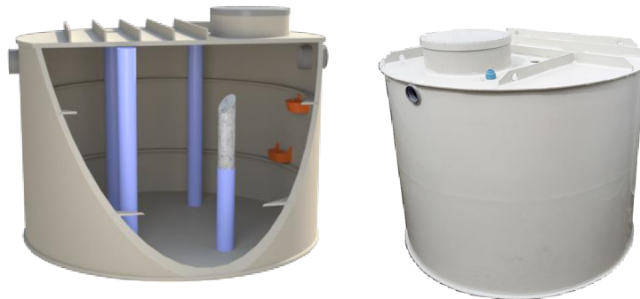
Obr. 37 - Akumulací nádrž [68]
