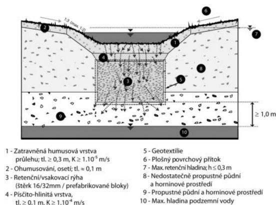
Obr. 13 - Vsakovací průleh-rýha [19]
