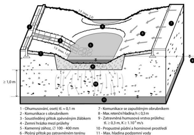
Obr. 12 - Vsakovací průleh [19]
