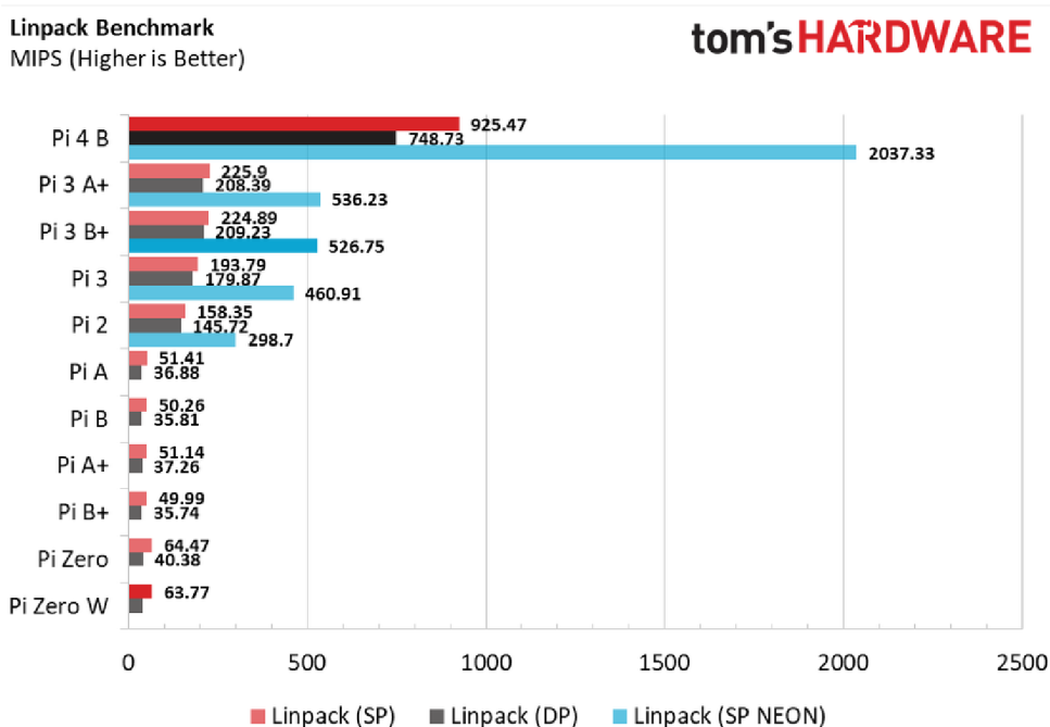
Obrázek 7 Linpack Benchmark (30)
