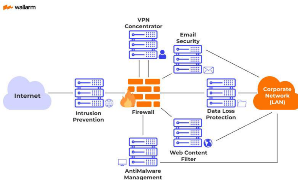
Obrázek 1 Diagram UTM (1)
